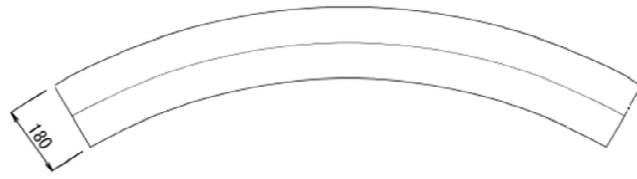
図-8-1 セグメント標準断面図（円周方向）（鉄筋コンクリート造）
