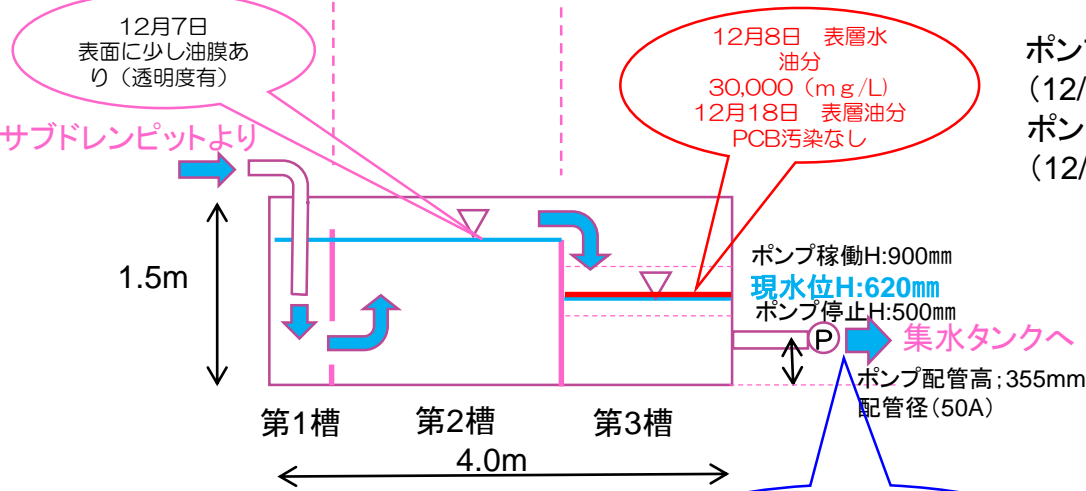
断面図
