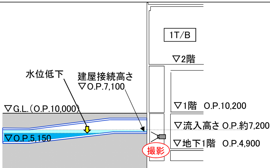
A-A断面図
