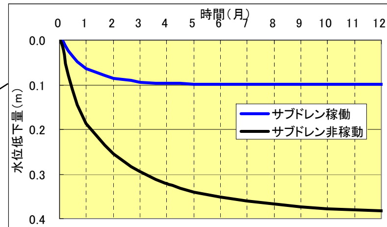
陸側遮水壁の遮水性発現後の地下水位の経時変化
