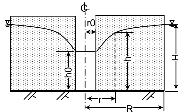
不圧帯水層の軸対象定常浸透流
