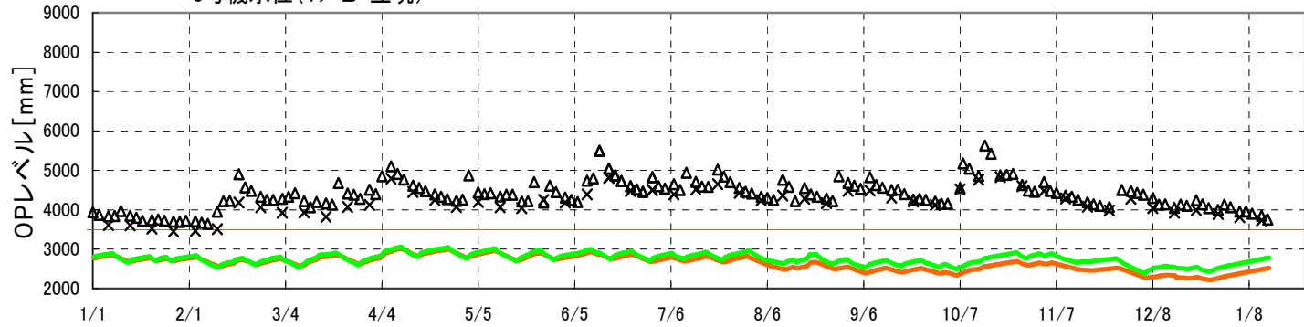
3号機水位(R/B)
