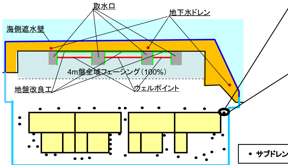
陸側遮水壁（山側3辺）
