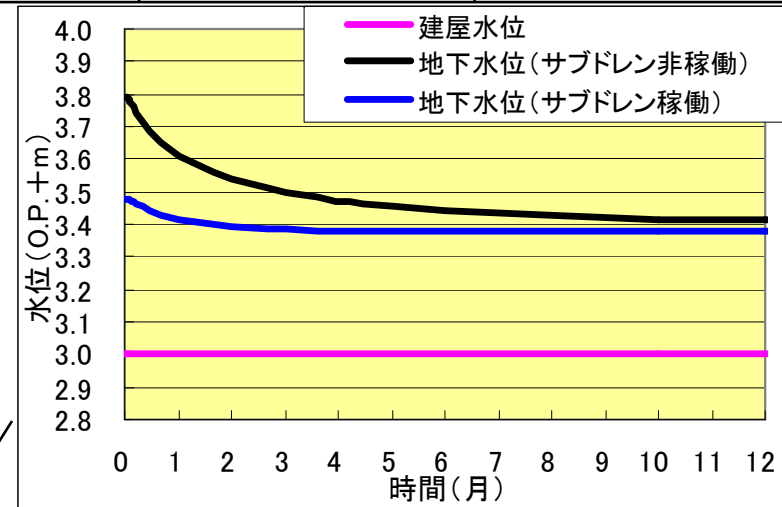
陸側遮水壁の遮水性発現後の地下水位の経時変化
