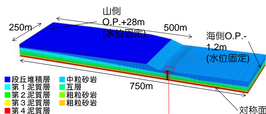
解析メッシュ図(1/2対称モデル)
