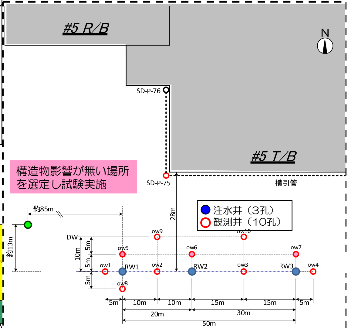
注水井・観測井配置図
