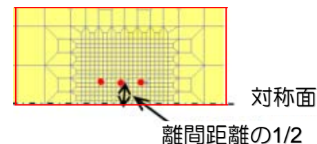
解析メッシュ拡大図(平面図)
