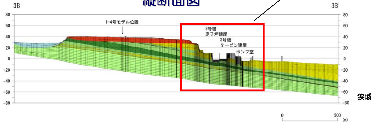
縦断面図
