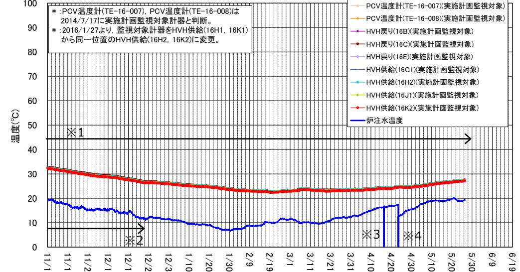
2号機 D/W雰囲気温度(11/1~5/26)
