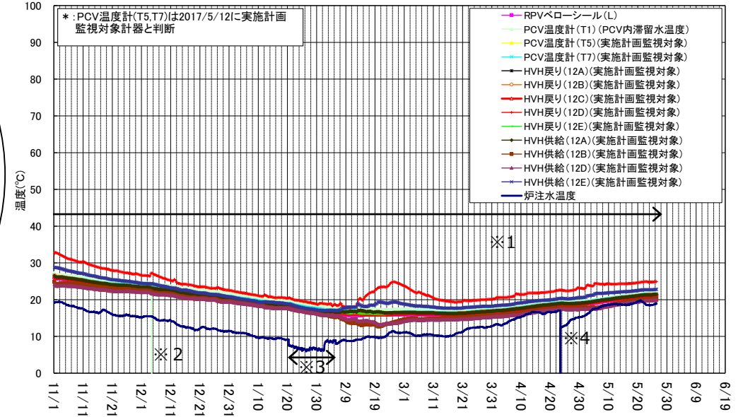
1号機 D/W雰囲気気温度 (11/1~5/26)
