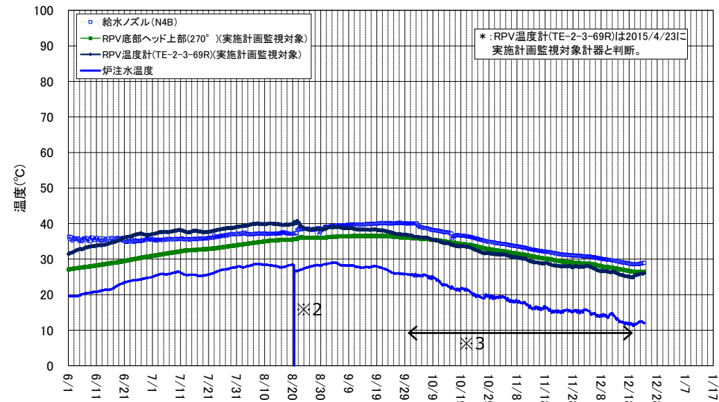
2号機 原子炉圧力容器まわり温度(6/1～12/23)
