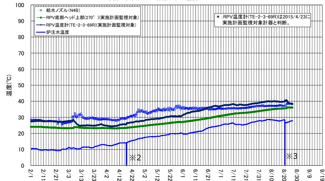
2号機 原子炉圧力容器まわり温度(2/1～8/26)
