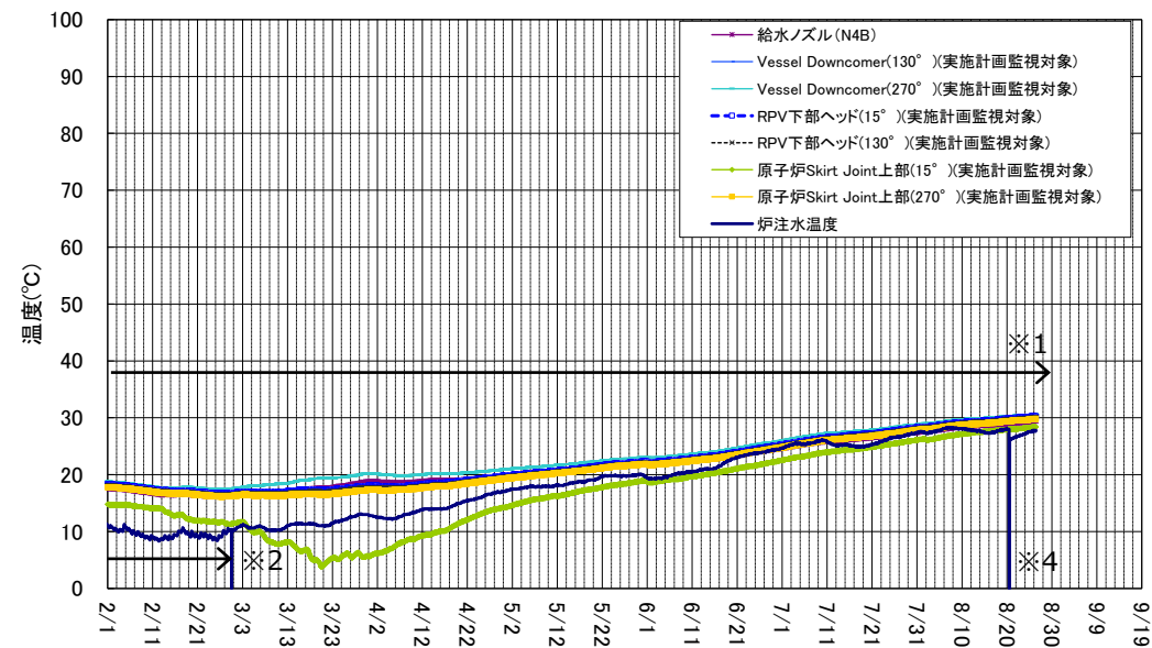
1号機 原子炉圧力容器まわり温度 (2/1~8/26)
