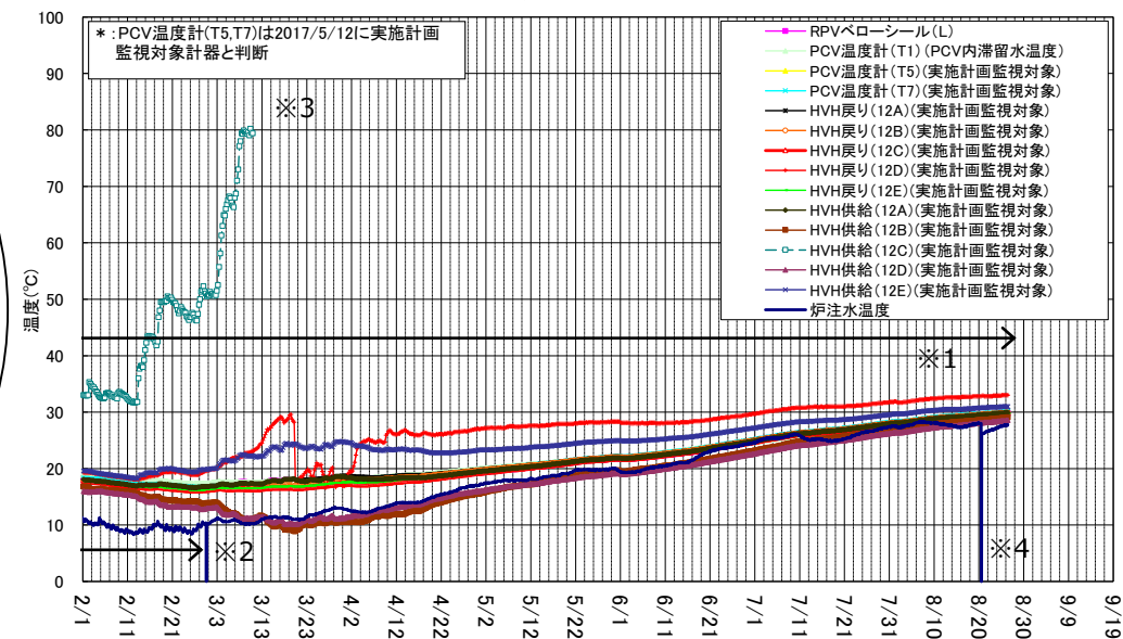
1号機 D/W雰囲気気温度 (2/1~8/26)
