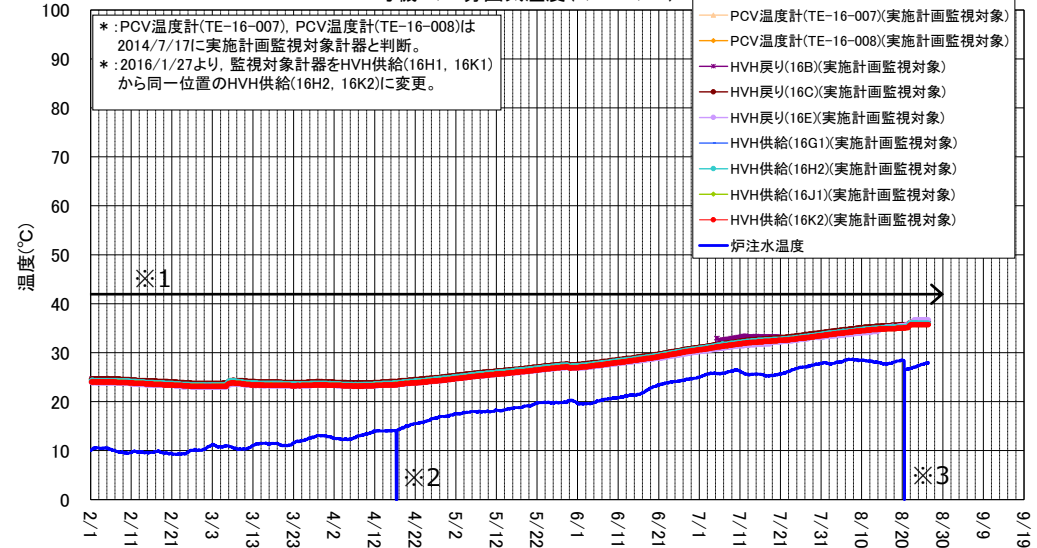
2号機 D/W雰囲気温度(2/1～8/26)
