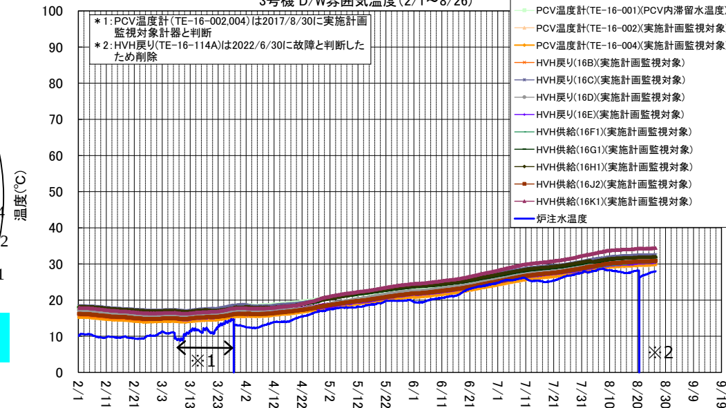
3号機 D/W雰囲気温度(2/1~8/26)
