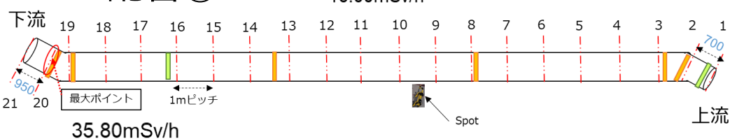
配管⑧
