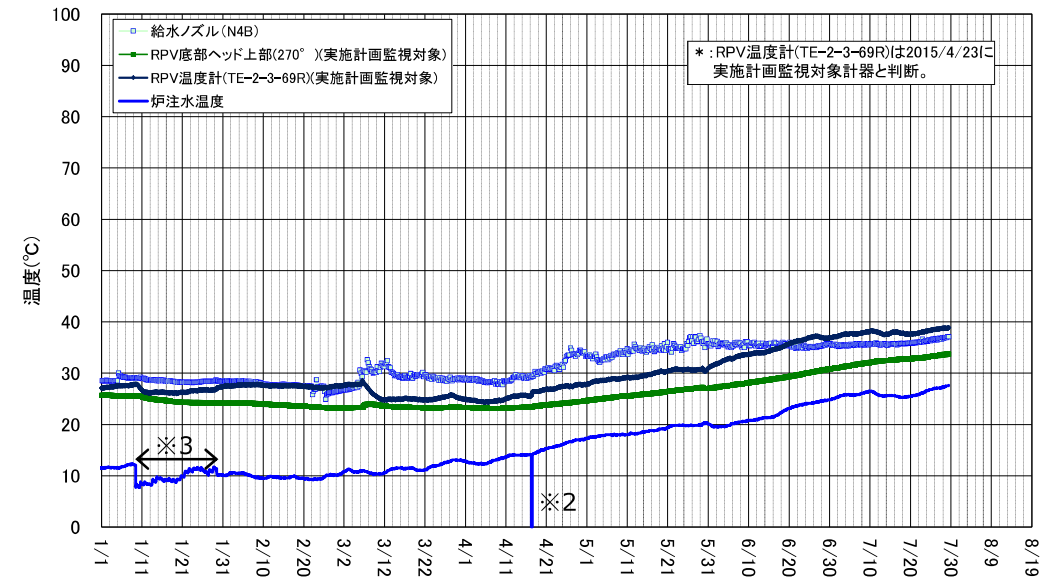
2号機 原子炉圧力容器まわり温度(1/1～7/29)
