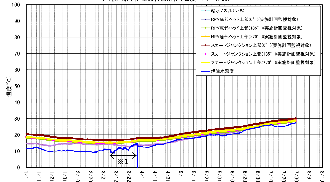
3号機 D/W雰囲気温度 (1/1～7/29)
