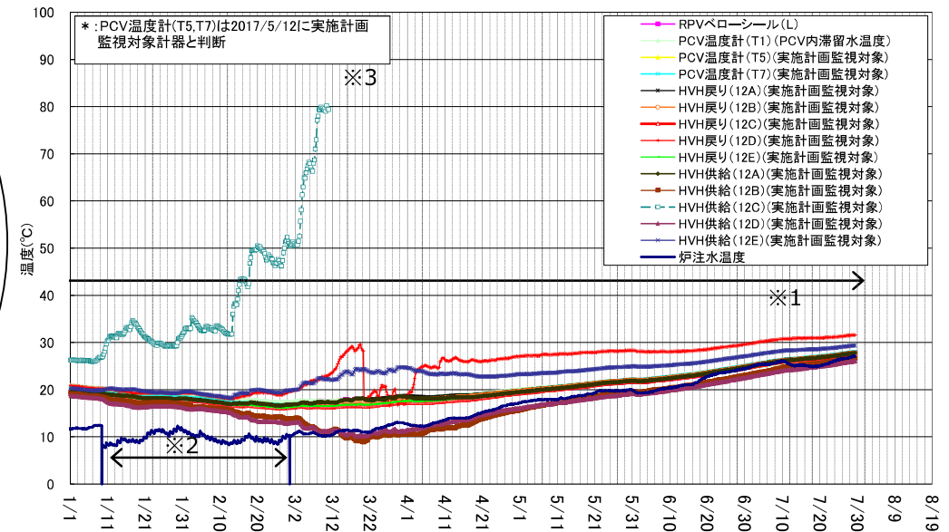
1号機 D/W雰囲気温度(1/1～7/29)
