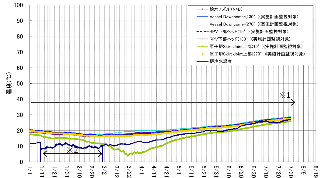
1号機 原子炉圧力容器まわり温度(1/1～7/29)
