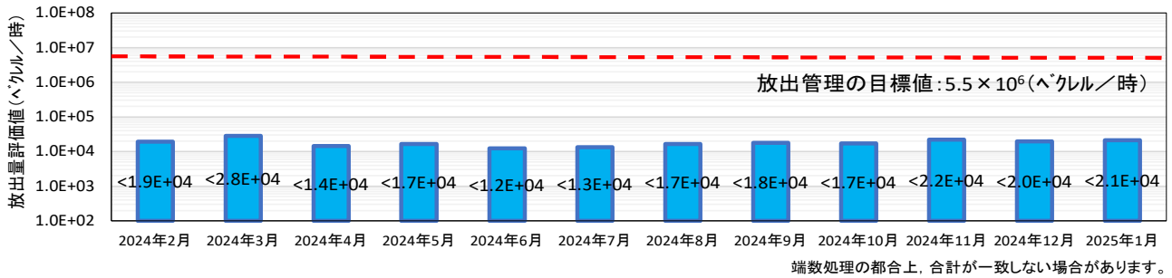
1号機 原子炉建屋, PCVガス管理システムからの放出量推移
