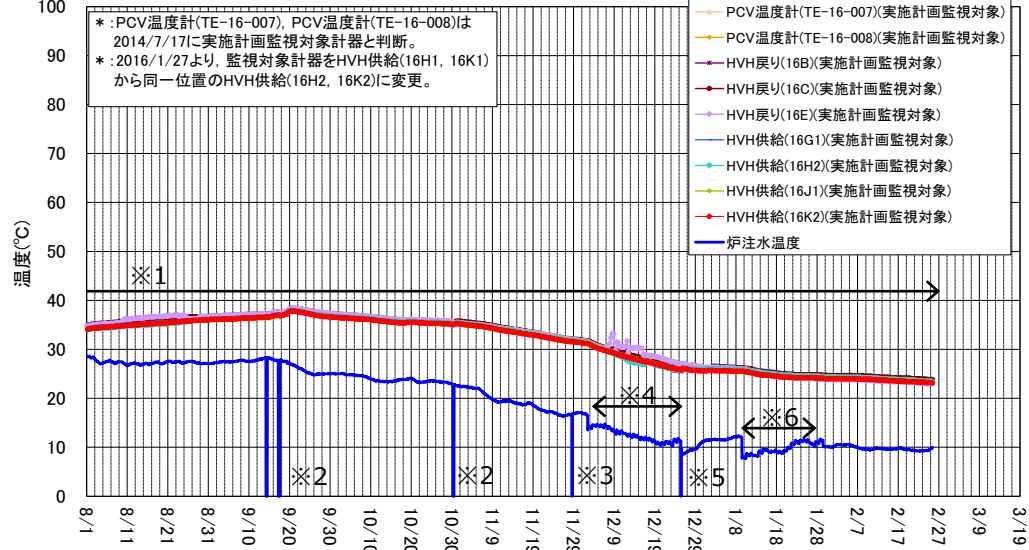
2号機 D/W雰囲気温度 (8/1~2/25)
