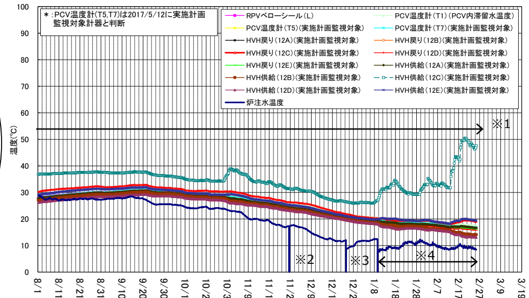
1号機 D/W雰囲気温度(8/1~2/25)
