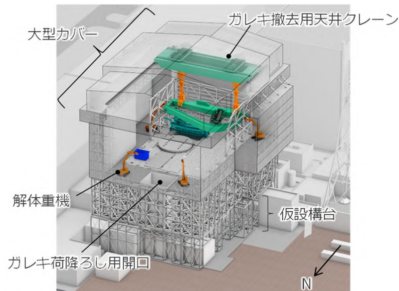
図 1号機 がれき撤去時（イメージ図）
