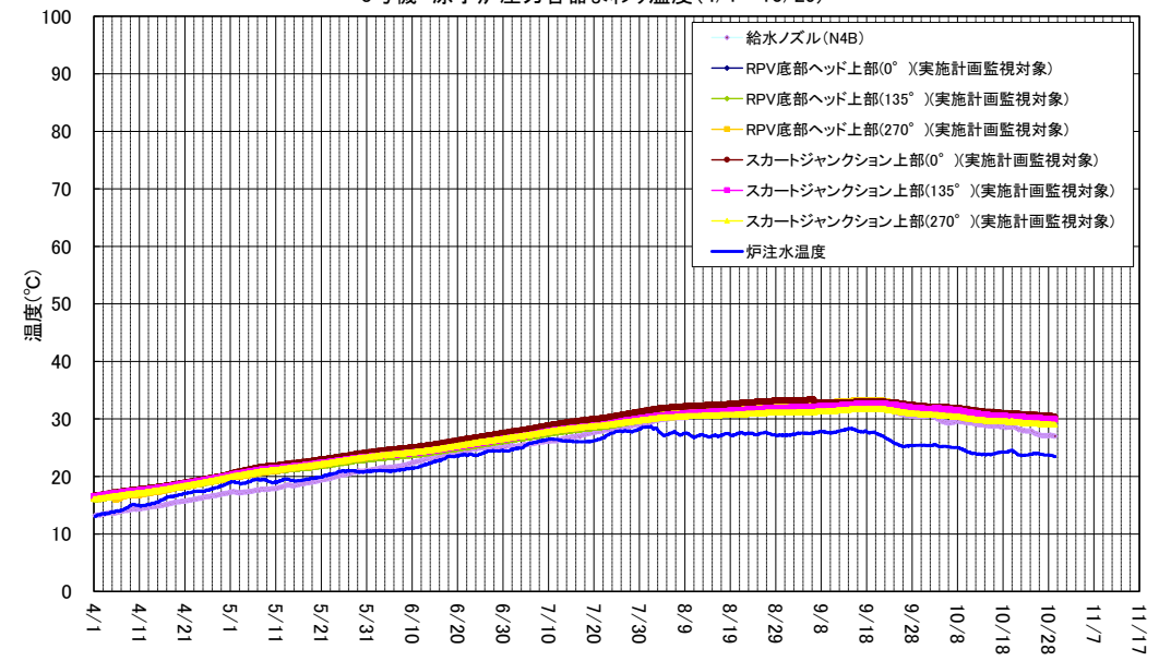
3号機 原子炉压力容器まわり温度 (4/1~10/29)
