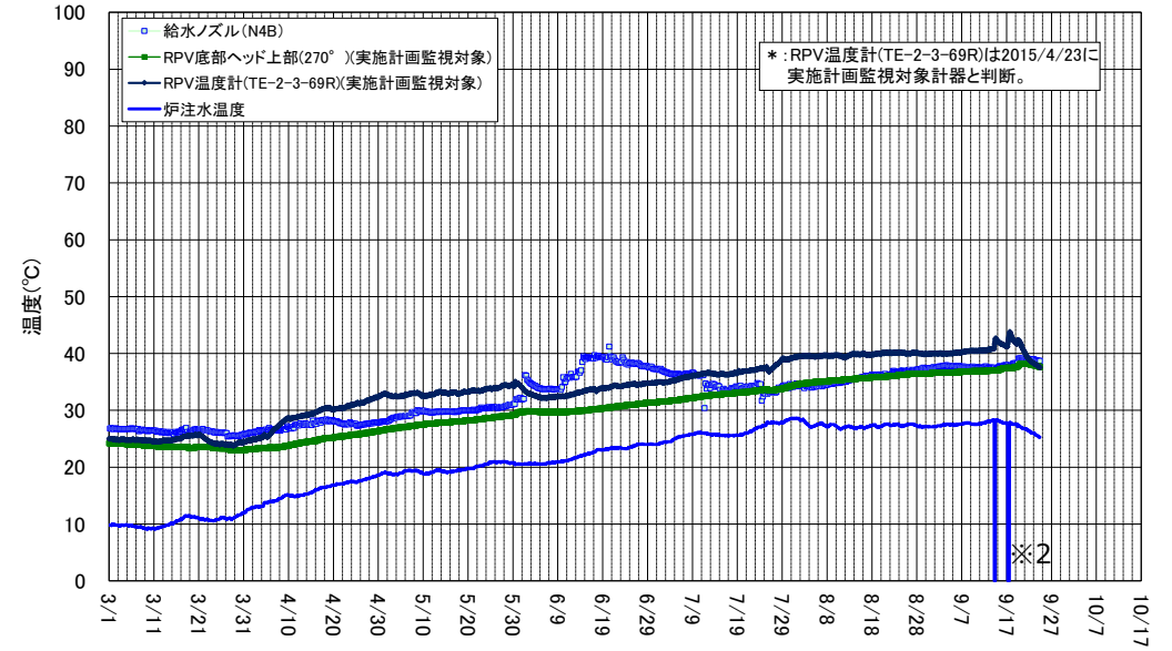
2号機 原子炉圧力容器まわり温度 (3/1~9/24)
