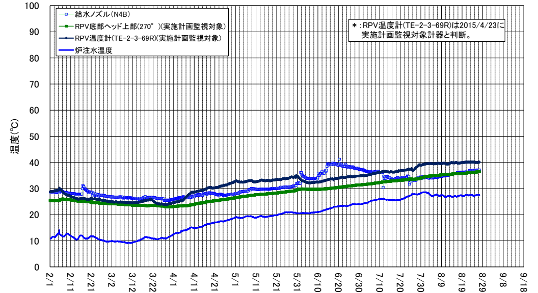
2号機 原子炉圧力容器まわり温度(2/1~8/27)
