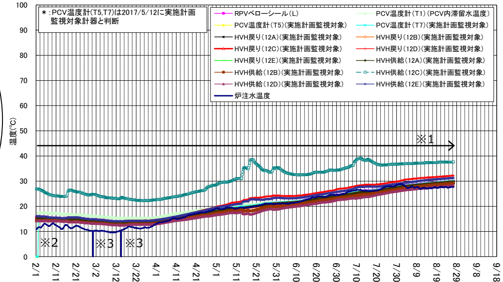
1号機 D/W雰囲気気温度(2/1~8/27)
