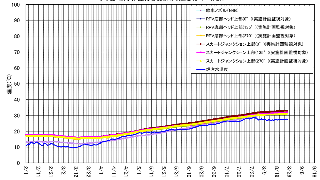
3号機 原子炉圧力容器まわり温度(2/1~8/27)
