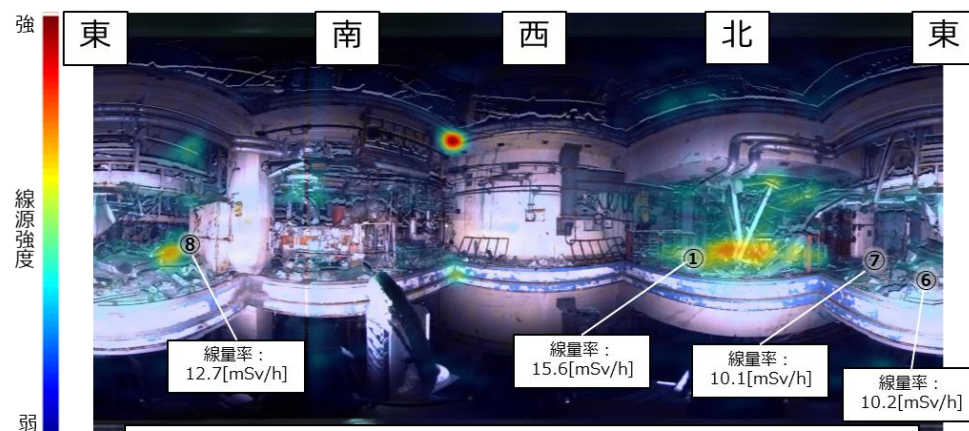
3号機R/B 3階 機器ハッチ近傍のγ線源強度分布
