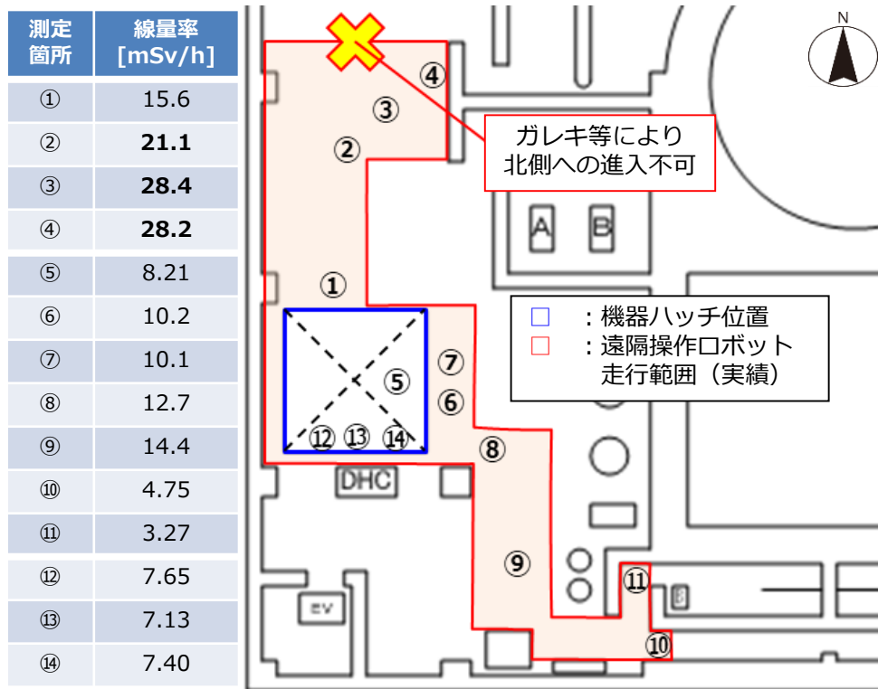
3号機R/B 3階 機器ハッチ近傍の空間線量率
