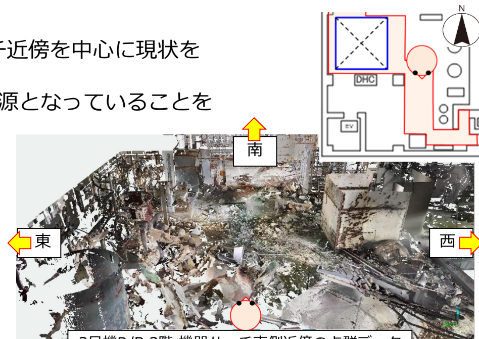
3号機R/B 3階 機器ハッチ東側近傍の点群データ
