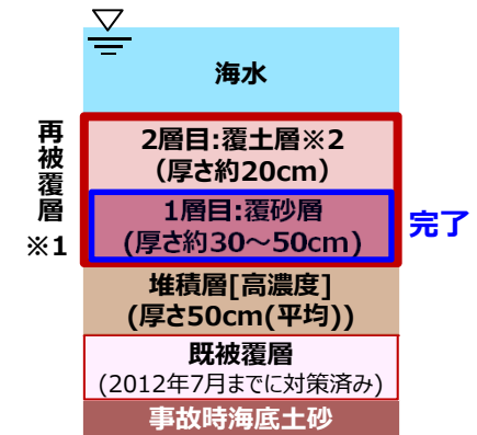
図11.層構成詳細
