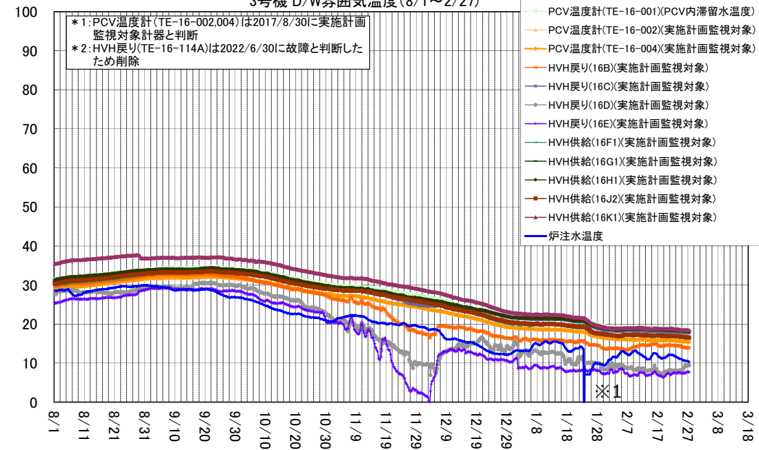
3号機 D/W雰囲気温度(8/1~2/27)
