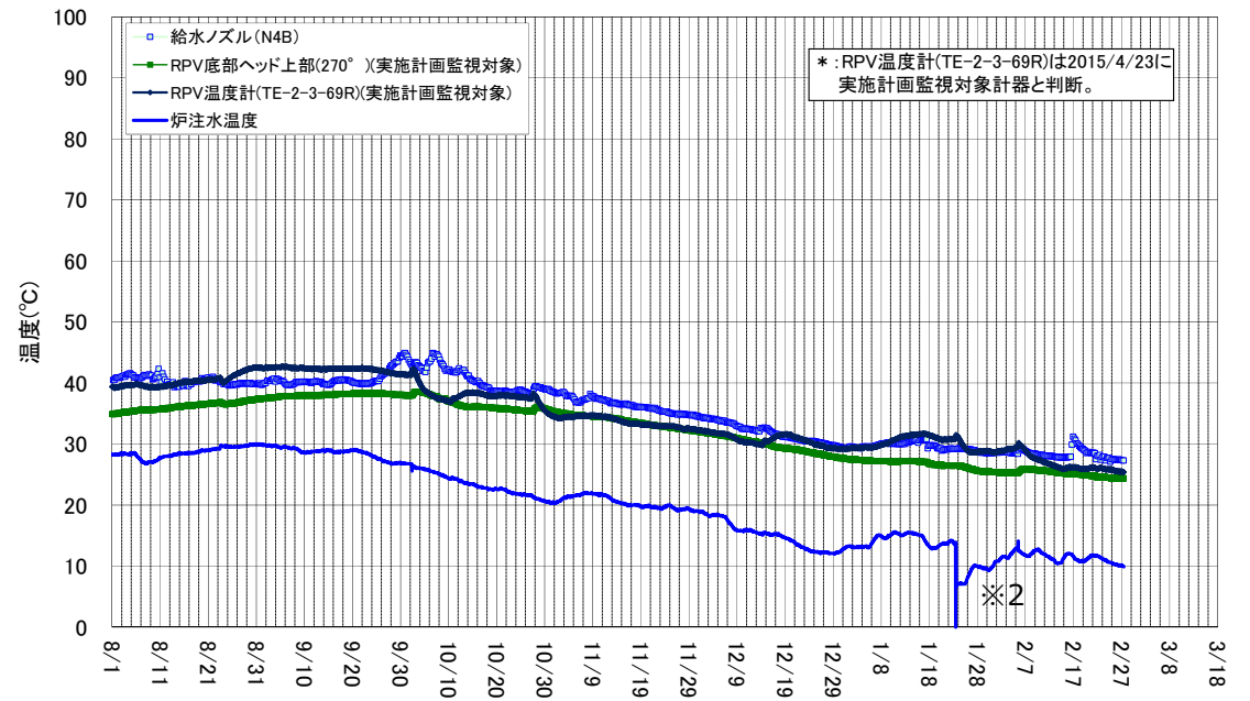
2号機 原子炉圧力容器まわり温度(8/1~2/27)
