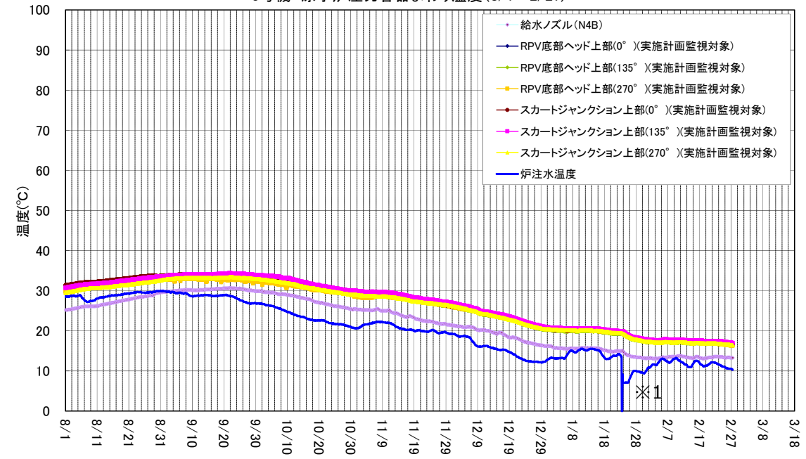
3号機 原子炉圧力容器まわり温度(8/1~2/27)
