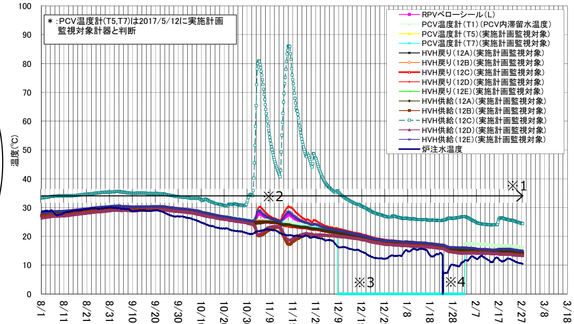
1号機 D/W雰囲気温度(8/1~2/27)
