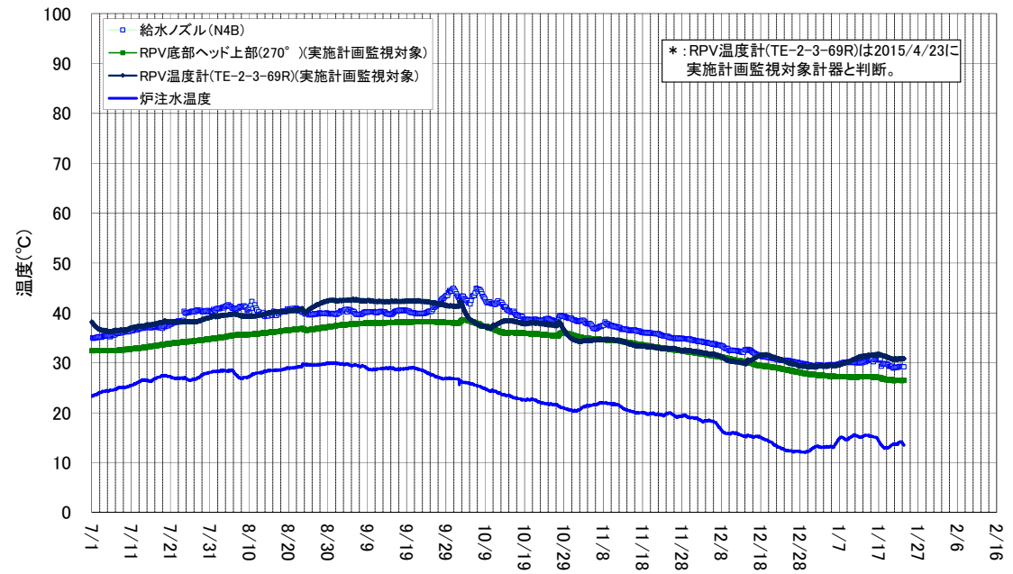
2号機 原子炉圧力容器まわり温度(7/1~1/23)
