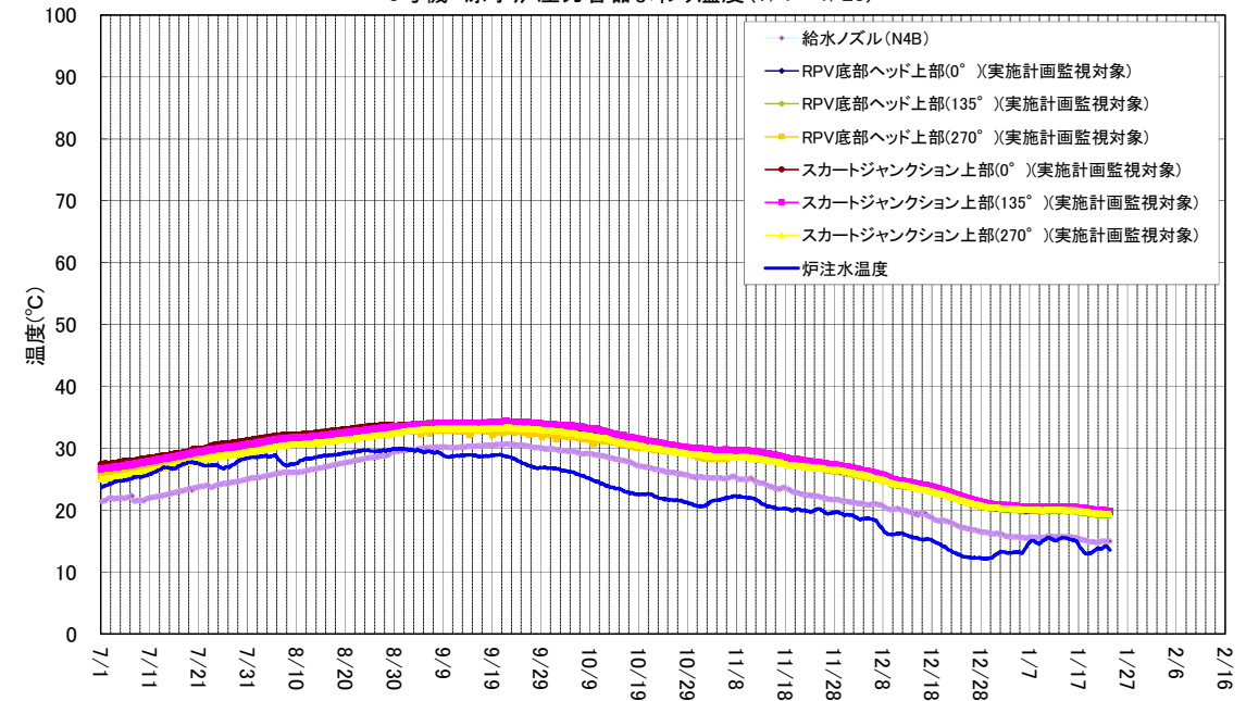
3号機 原子炉压力容器まわり温度 (7/1~1/23)
