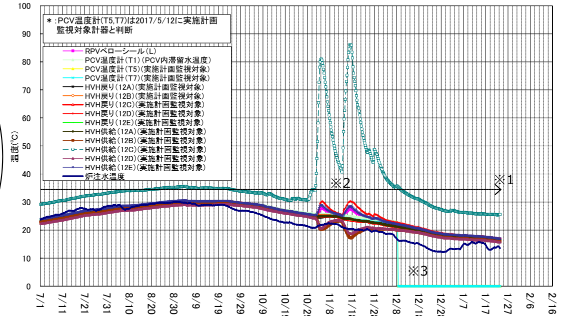
1号機 D/W雰囲気温度(7/1~1/23)
