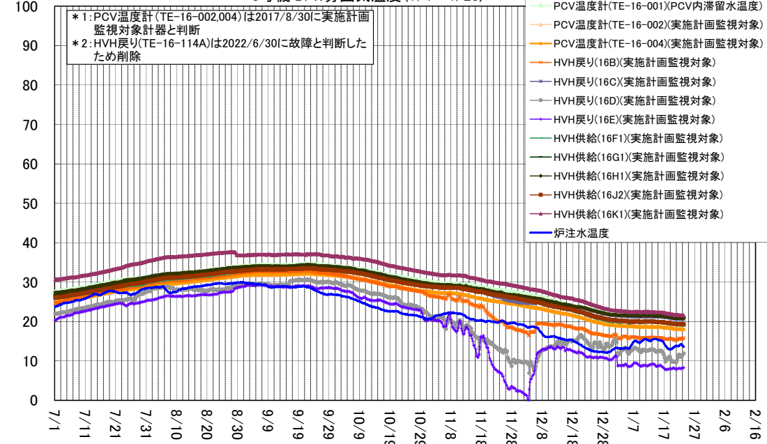
3号機 D/W雰囲気温度 (7/1~1/23)
