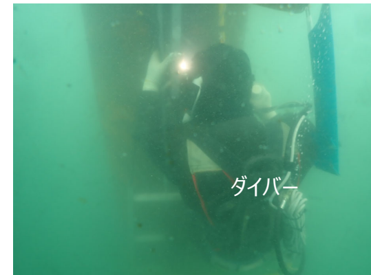
取り付けガイド設置（溶接）
