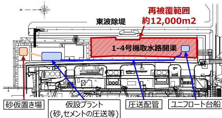
再被覆工事概要図
