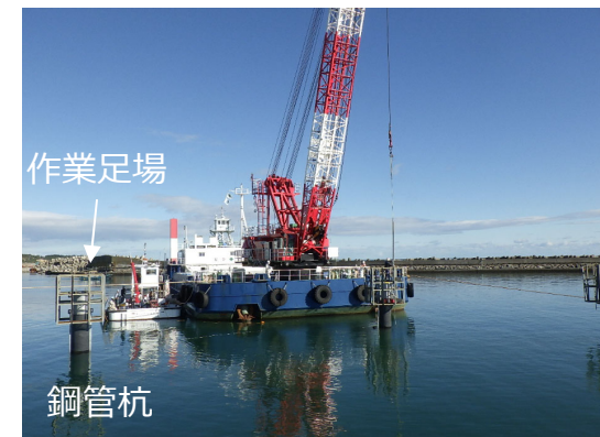
取り付けガイド設置（吊り上げ）
