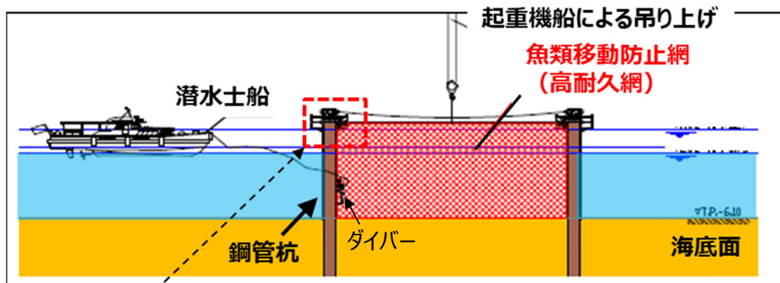
高耐久網取付方法
