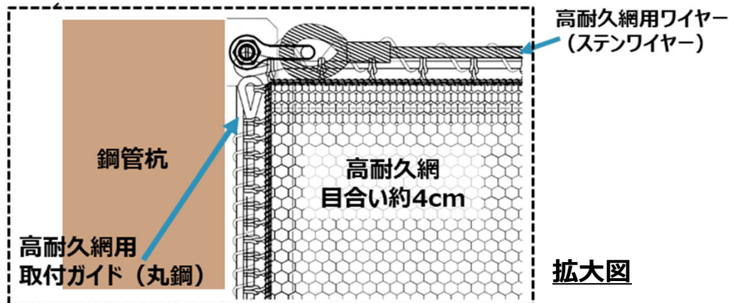
高耐久網取付方法
