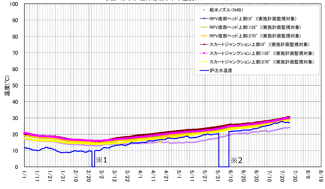
3号機 原子炉压力容器まわり温度(1/1~7/25)
