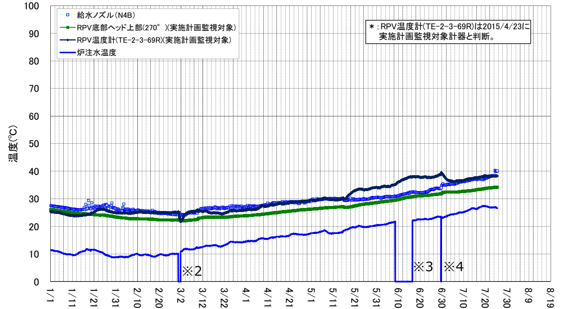
2号機 原子炉圧力容器まわり温度(1/1~7/25)
