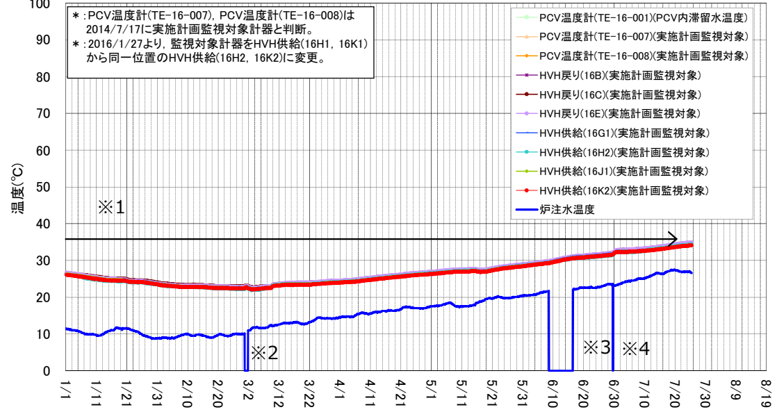
2号機 D/W雰囲気温度(1/1~7/25)
