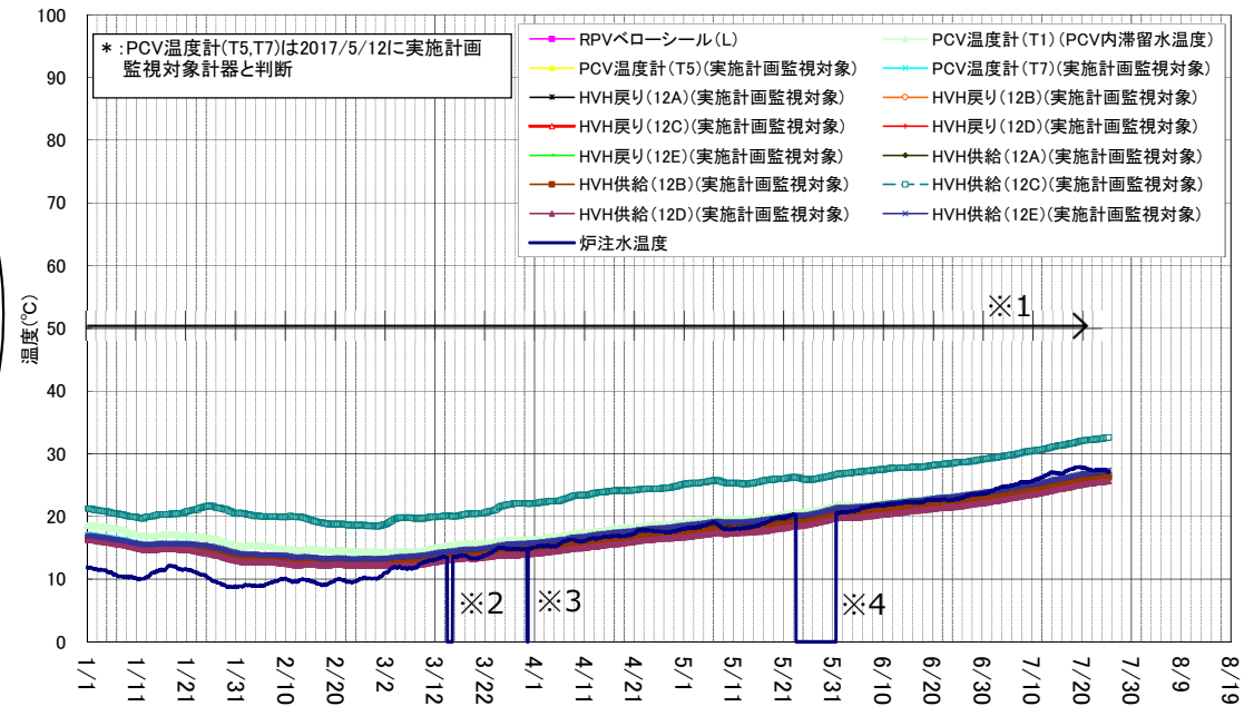
1号機 D/W雰囲気温度(1/1~7/25)
