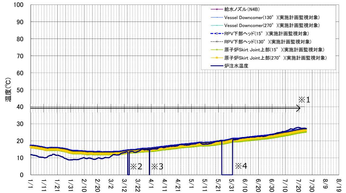
1号機 原子炉圧力容器まわり温度(1/1~7/25)
