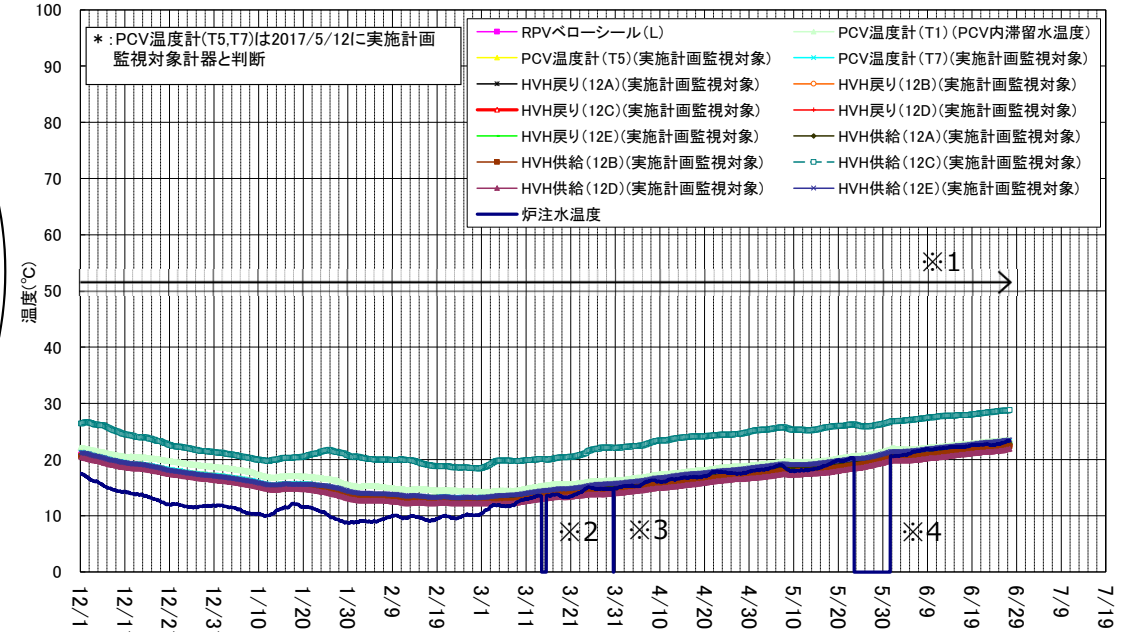
1号機 D/W雰囲気温度(12/1~6/27)
