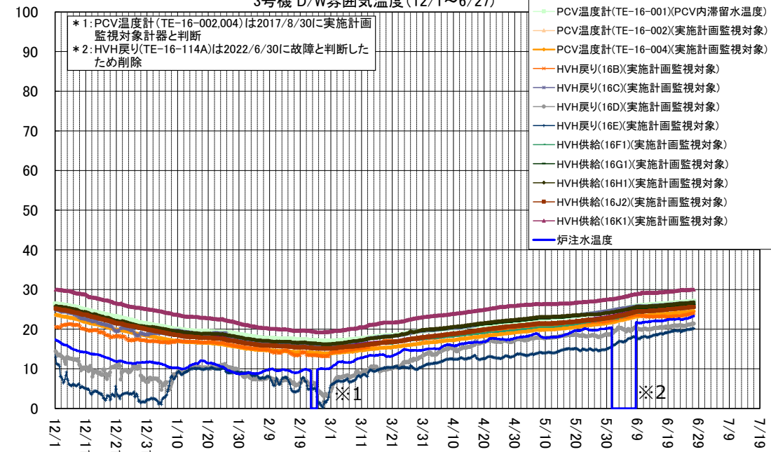
3号機 D/W雰囲気温度(12/1~6/27)
