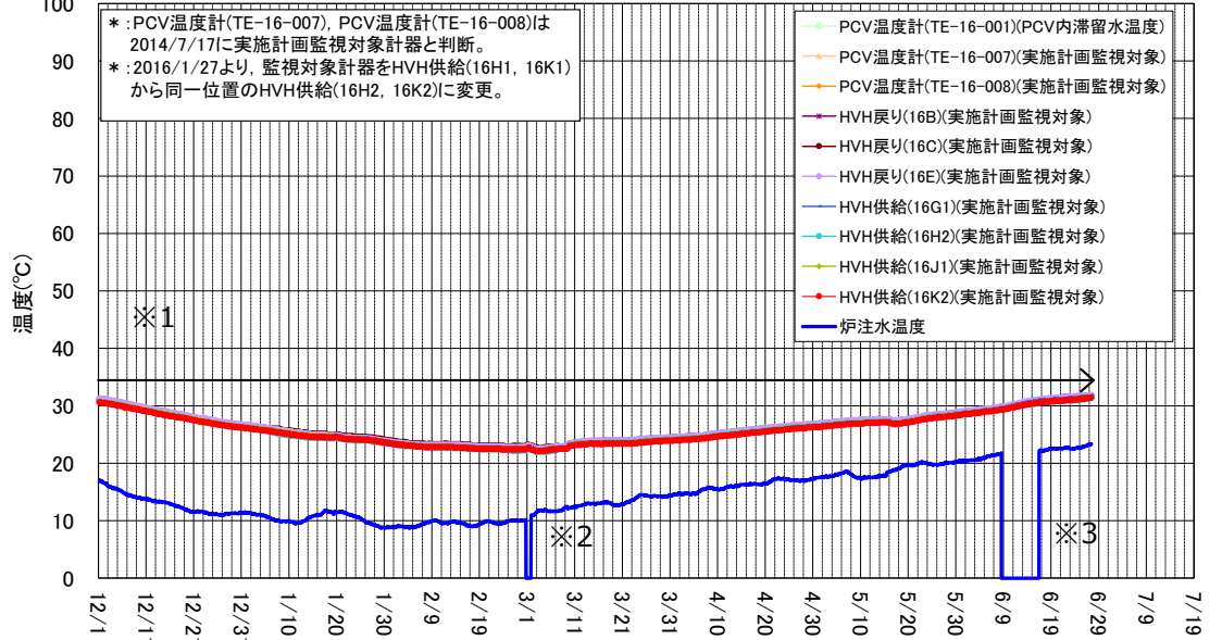
2号機 D/W雰囲気温度(12/1~6/27)
