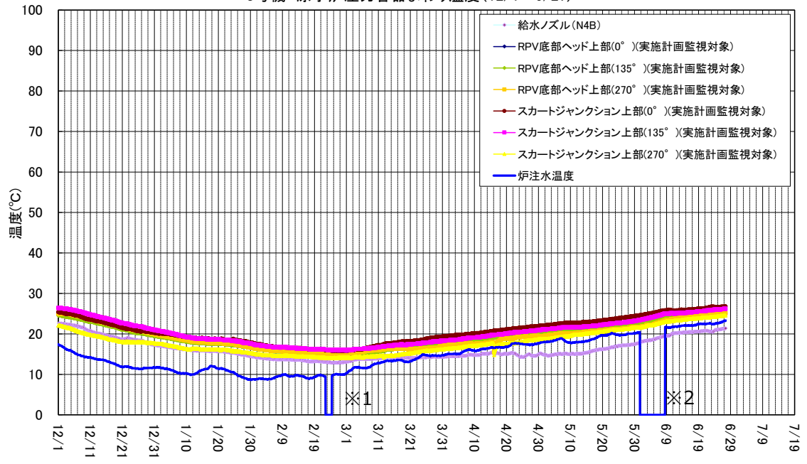
3号機 原子炉压力容器まわり温度(12/1~6/27)
