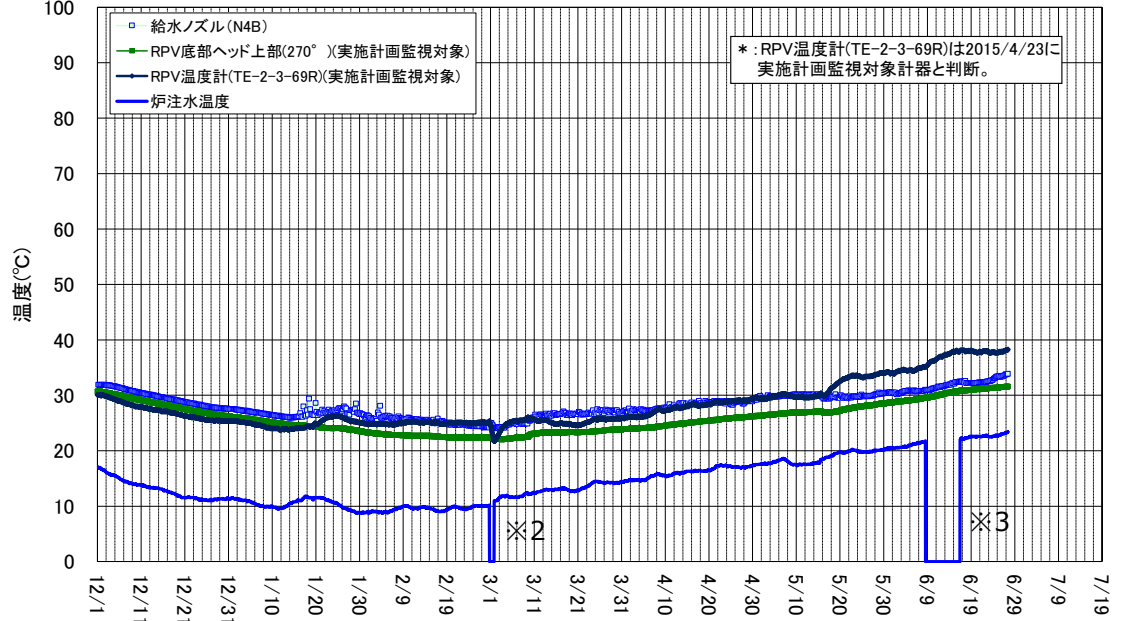
2号機 原子炉压力容器まわり温度(12/1~6/27)
