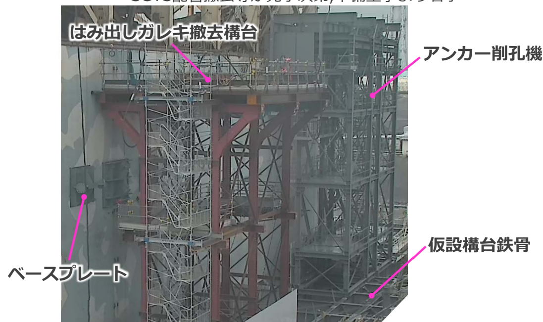
アンカー削孔状況（東面） (撮影：2023年5月15日)
