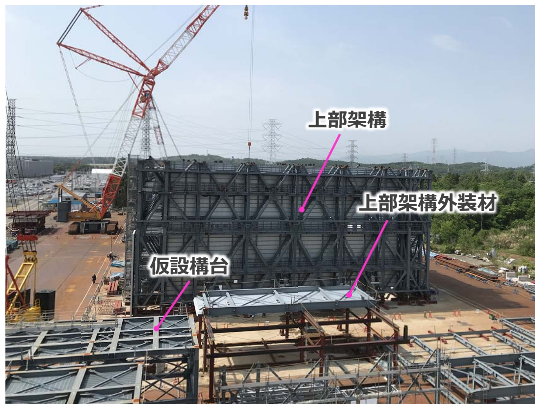
構外ヤード全景（撮影：2023年5月22日）
