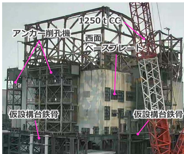
現場状況（北西面） (撮影：2023年5月23日)
