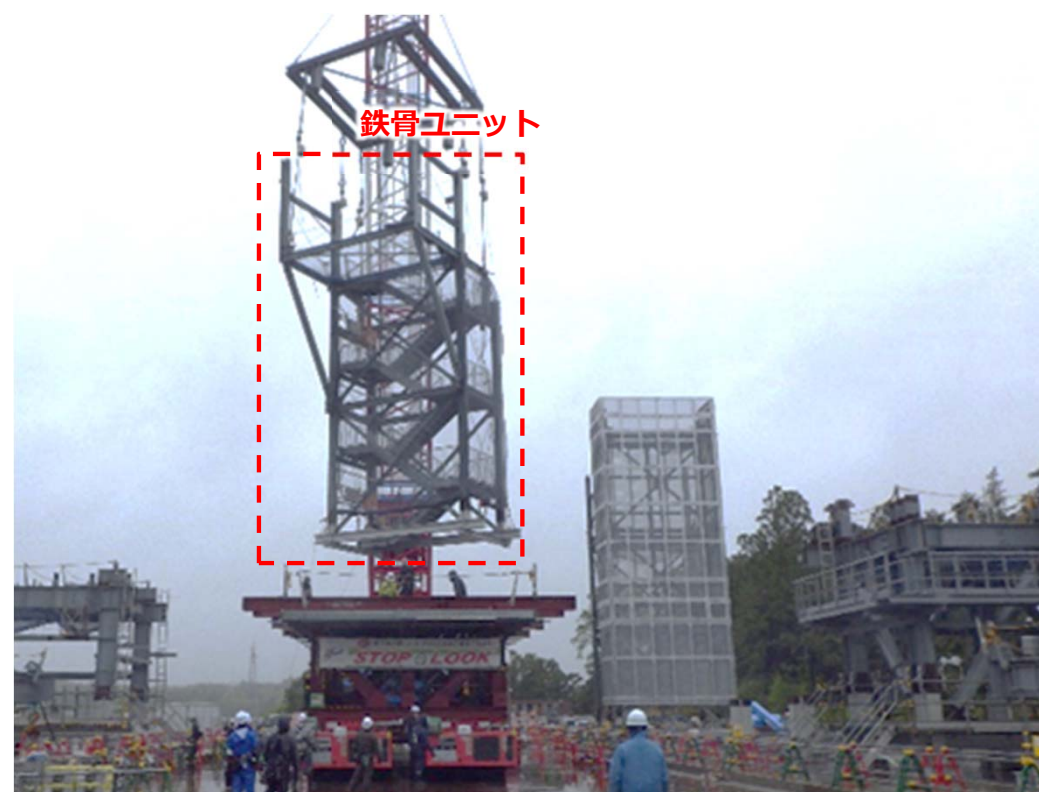
鉄骨ユニット運搬の実施状況（撮影：2023.4.26）
