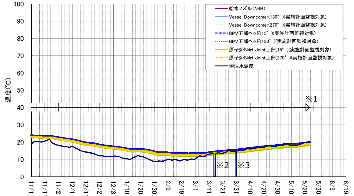
1号機 原子炉圧力容器まわり温度(11/1~5/23)
