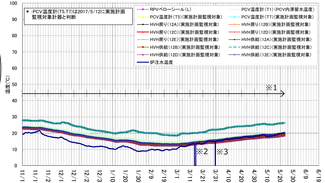
1号機 D/W雰囲気温度(11/1~5/23)
