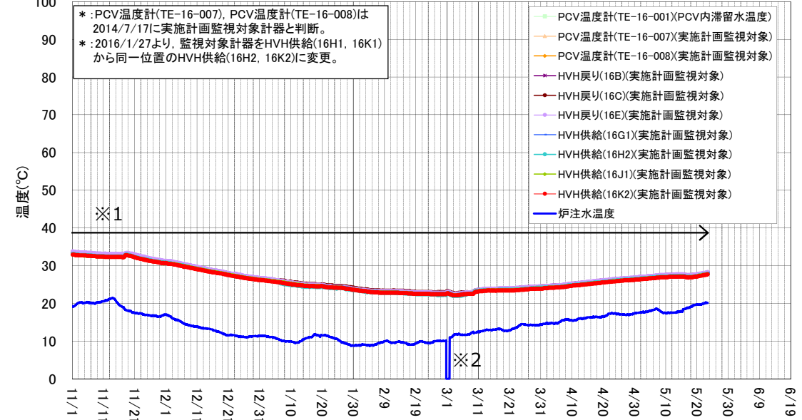
2号機 D/W雰囲気温度(11/1~5/23)
