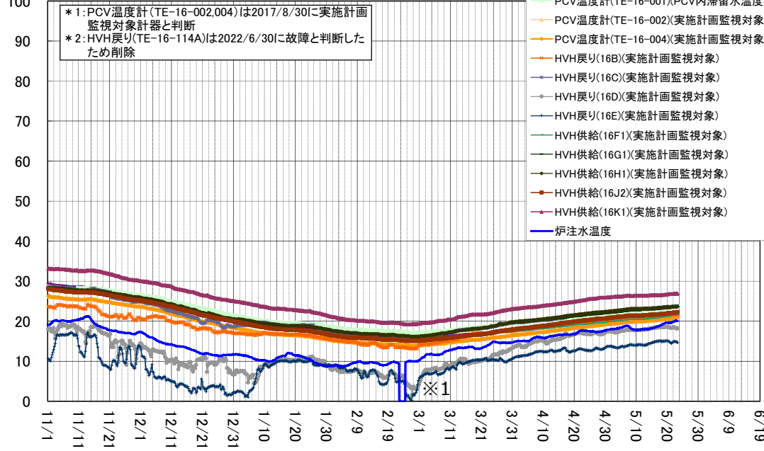
3号機 D/W雰囲気温度 (11/1~5/23)
