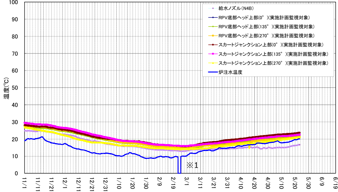
3号機 原子炉压力容器まわり温度 (11/1~5/23)
