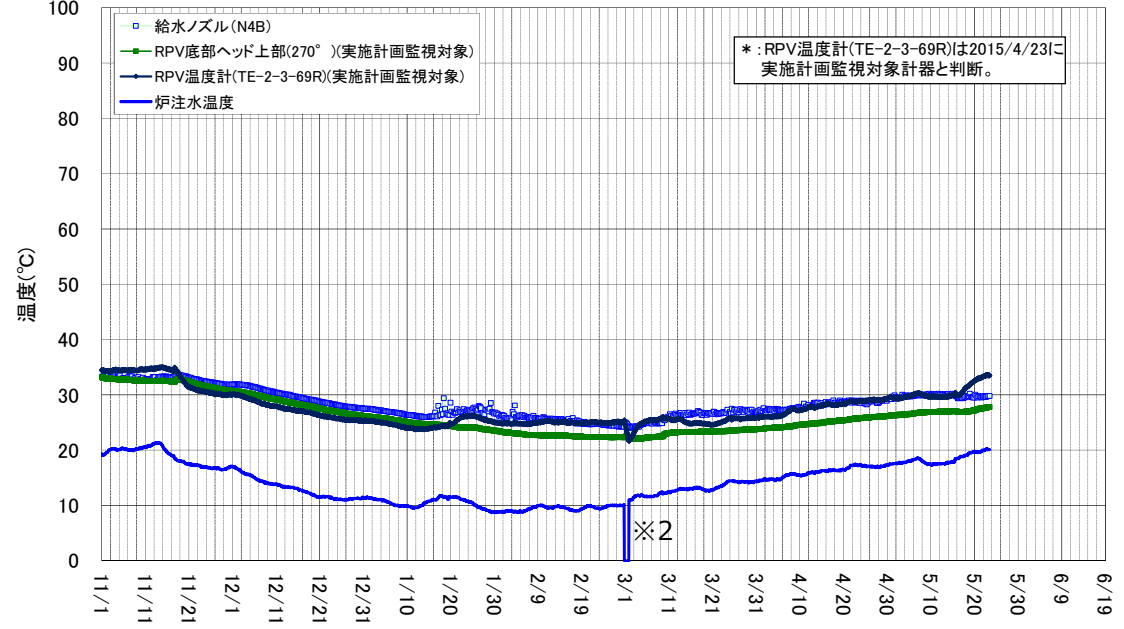
2号機 原子炉圧力容器まわり温度(11/1~5/23)
