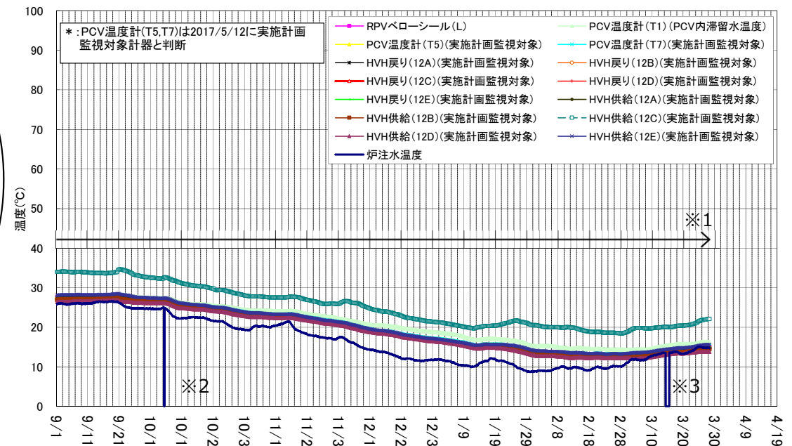
1号機 D/W雰囲気温度(9/1~3/28)
