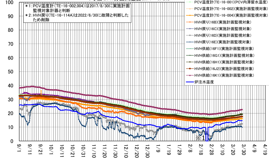
3号機 D/W雰囲気温度(9/1~3/28)
