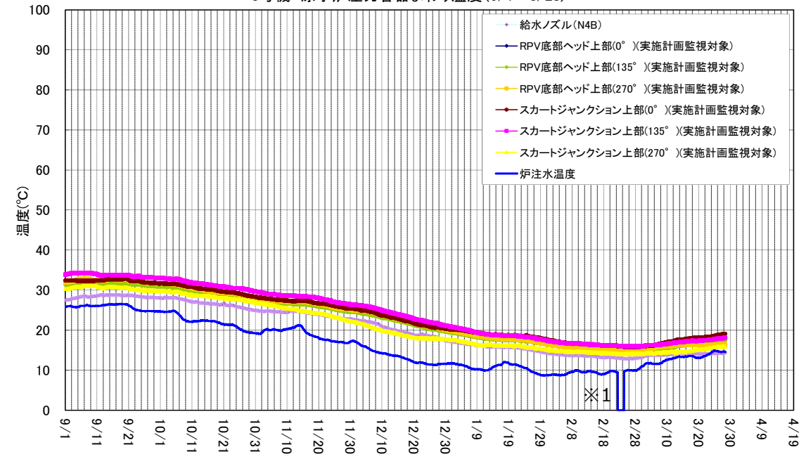
3号機 原子炉压力容器まわり温度(9/1~3/28)
