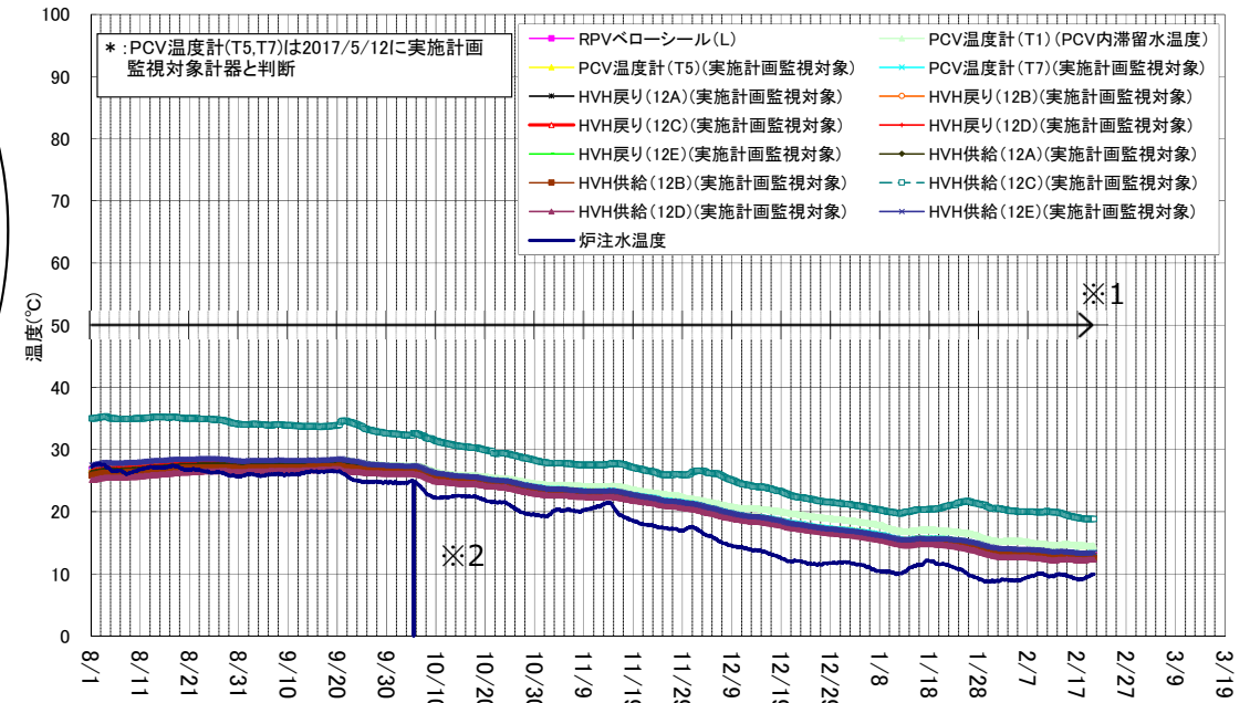
1号機 D/W雰囲気温度(8/1~2/20)
