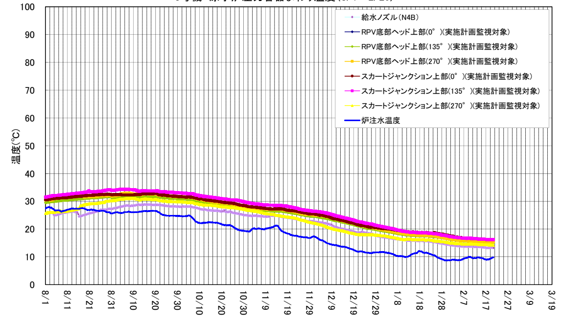
3号機 原子炉压力容器まわり温度(8/1~2/20)
