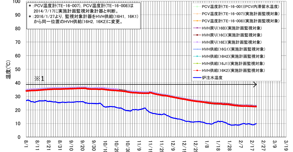
2号機 D/W雰囲気温度 (8/1~2/20)
