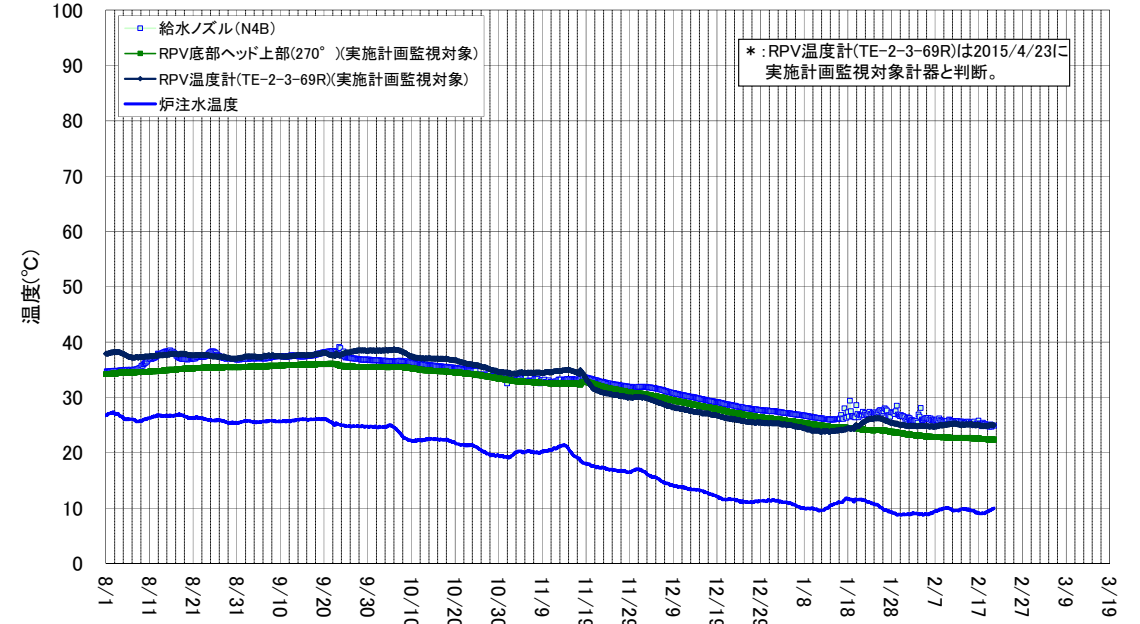
2号機 原子炉圧力容器まわり温度 (8/1~2/20)
