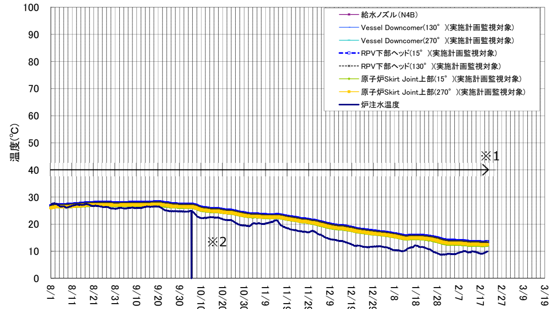
1号機 原子炉圧力容器まわり温度(8/1~2/20)
