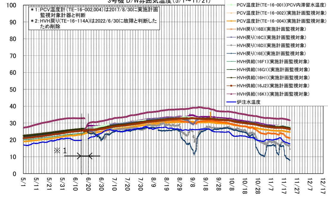
3号機 D/W雰囲気温度(5/1~11/21)
