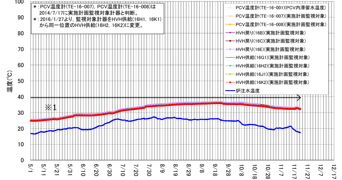
2号機 D/W雰囲気温度(5/1~11/21)
