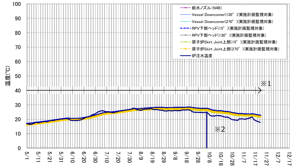
1号機 原子炉压力容器まわり温度(5/1~11/21)
