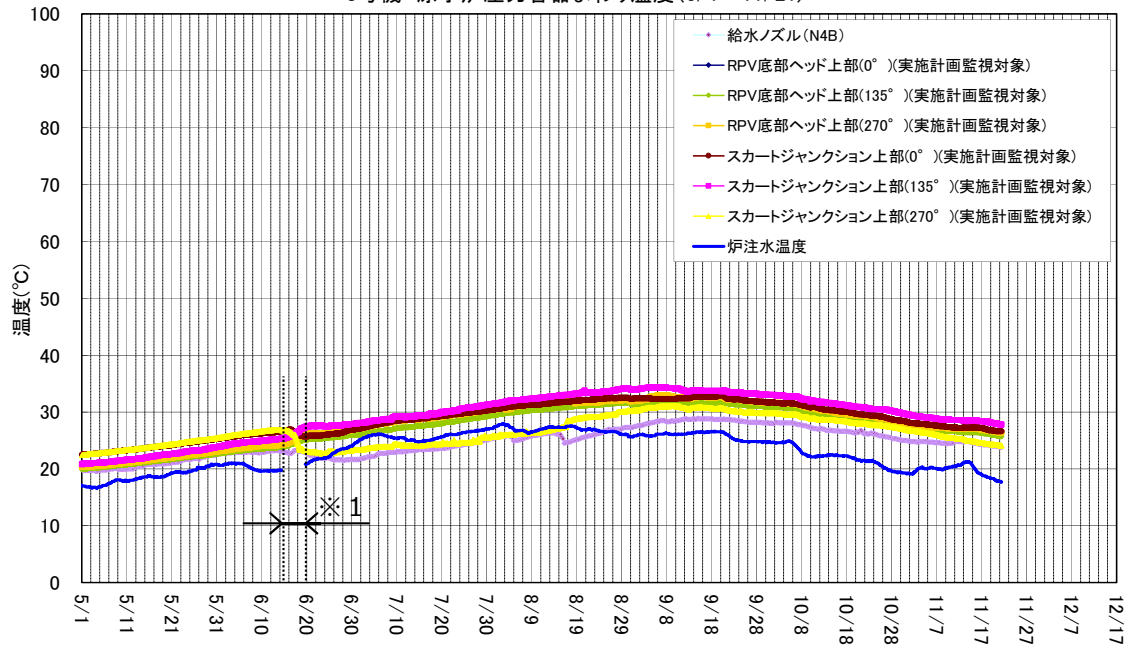
3号機 原子炉压力容器まわり温度(5/1~11/21)
