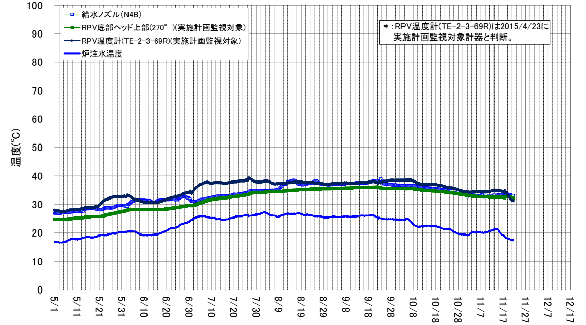
2号機 原子炉圧力容器まわり温度(5/1~11/21)
