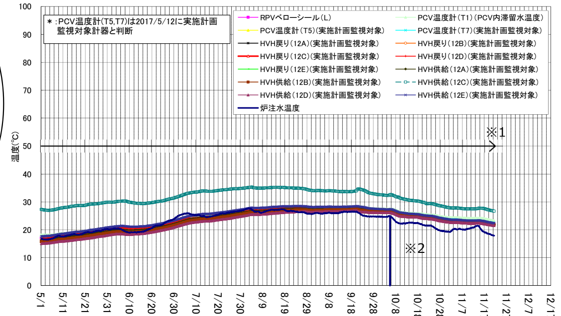
1号機 D/W雰囲気温度(5/1~11/21)
