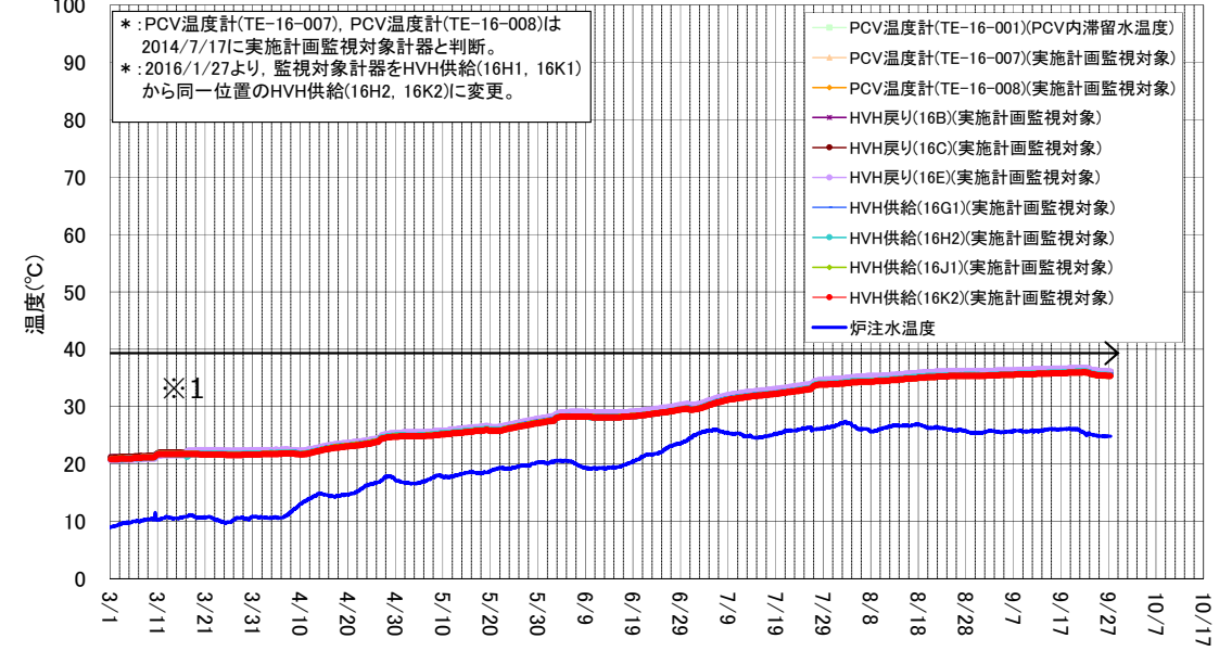
2号機 D/W雰囲気温度(3/1~9/27)
