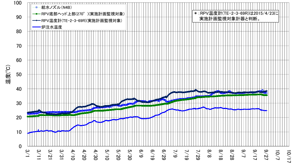
2号機 原子炉圧力容器まわり温度(3/1~9/27)
