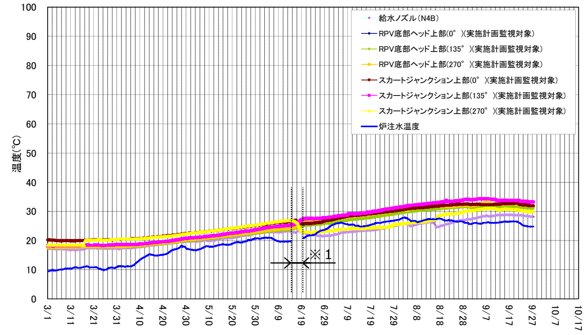
3号機 原子炉压力容器まわり温度(3/1~9/27)
