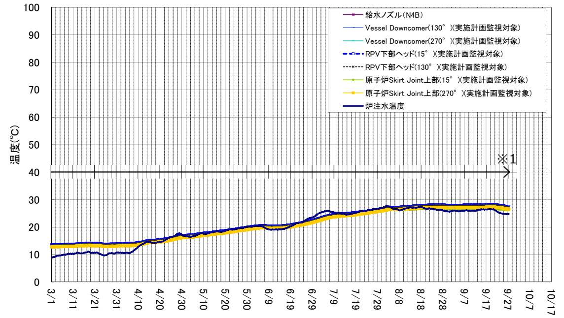
1号機 原子炉压力容器まわり温度(3/1~9/27)
