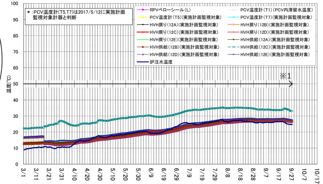
1号機 D/W雰囲気温度(3/1~9/27)
