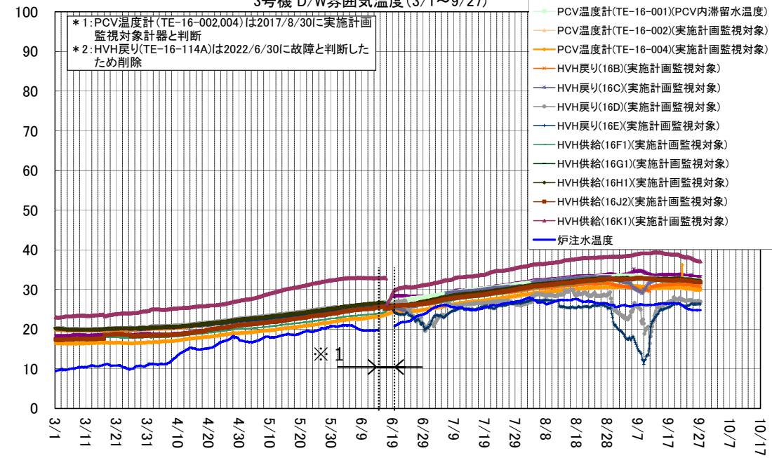
3号機 D/W雰囲気温度(3/1~9/27)
