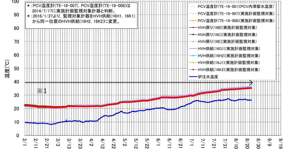
2号機 D/W雰囲気温度(2/1~8/23)
