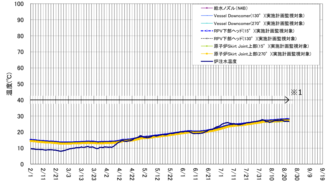
1号機 原子炉压力容器まわり温度(2/1~8/23)
