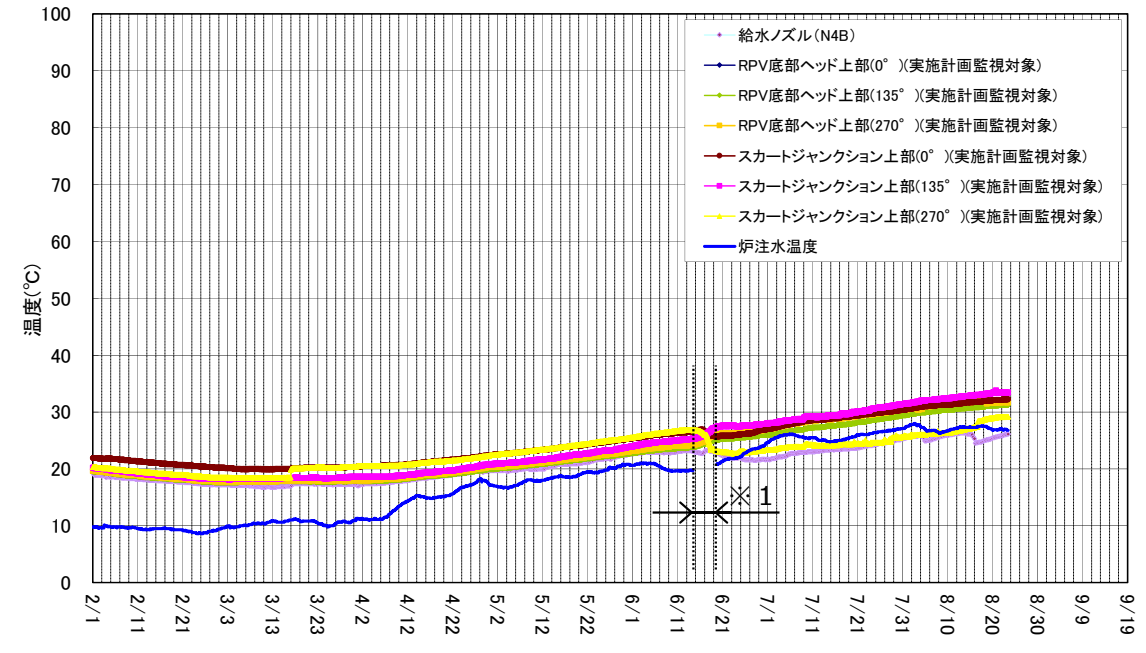
3号機 原子炉压力容器まわり温度 (2/1~8/23)
