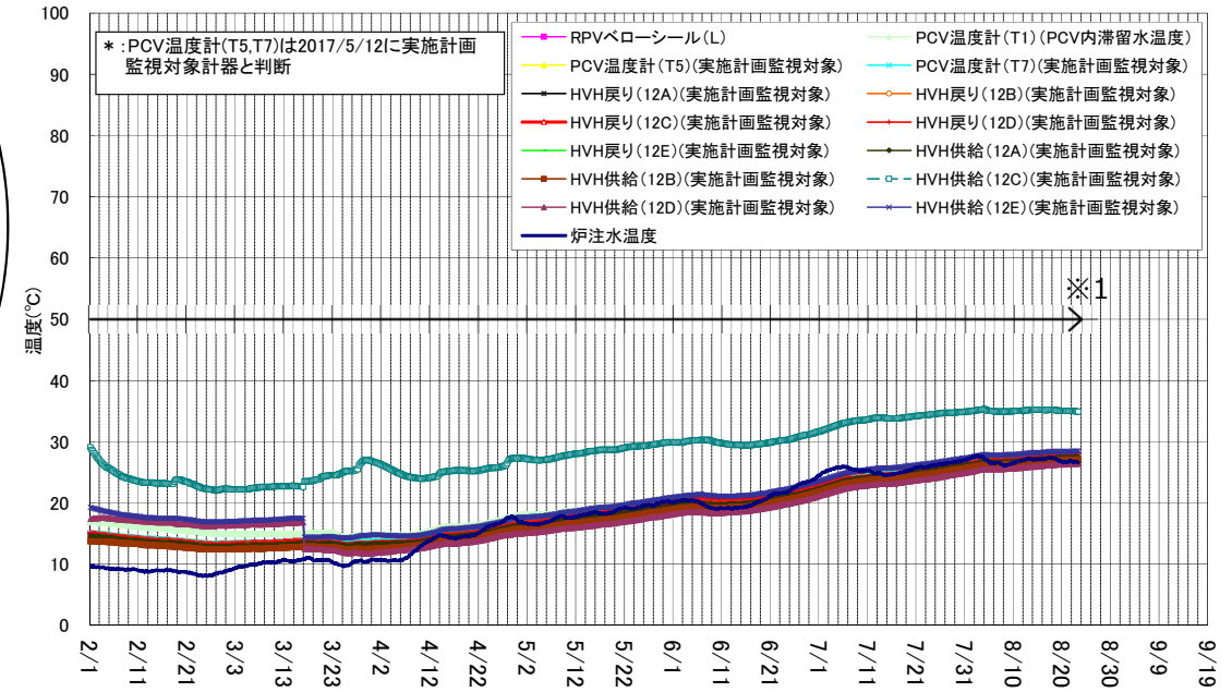
1号機 D/W雰囲気温度(2/1~8/23)
