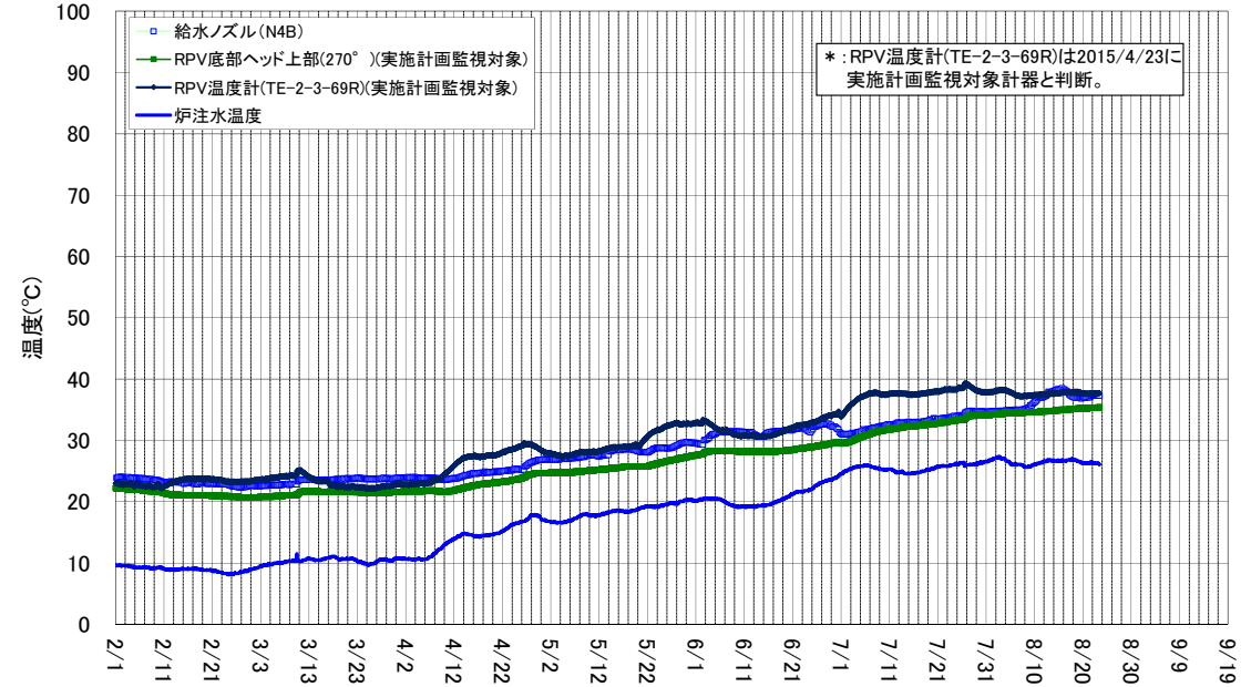
2号機 原子炉压力容器まわり温度(2/1~8/23)
