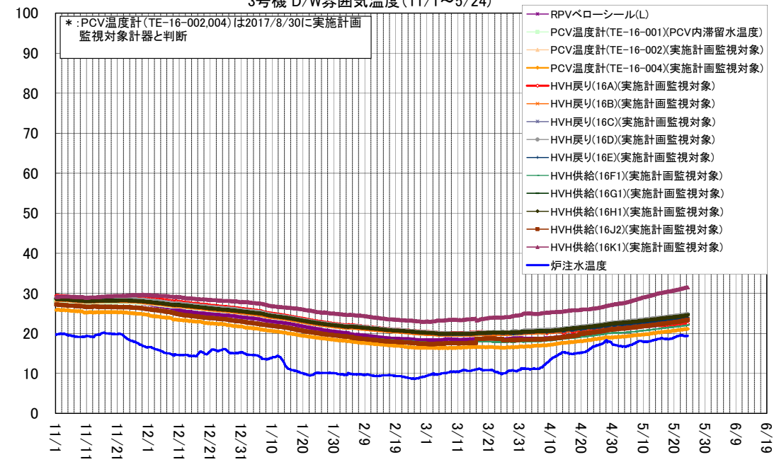
3号機 D/W雰囲気温度(11/1~5/24)
