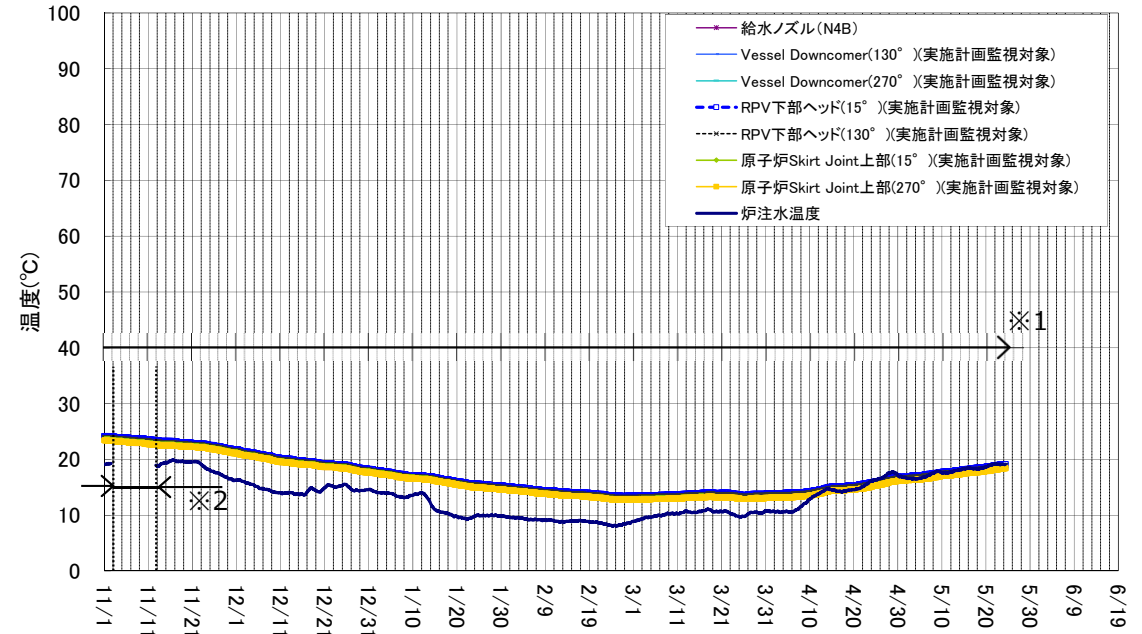
1号機 原子炉压力容器まわり温度(11/1~5/24)
