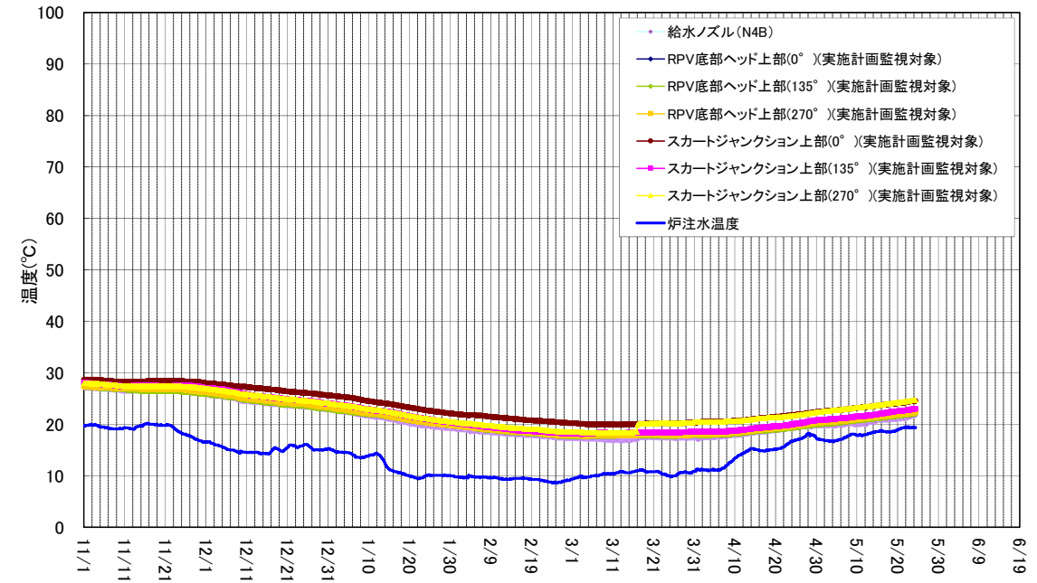
3号機 原子炉压力容器まわり温度(11/1~5/24)
