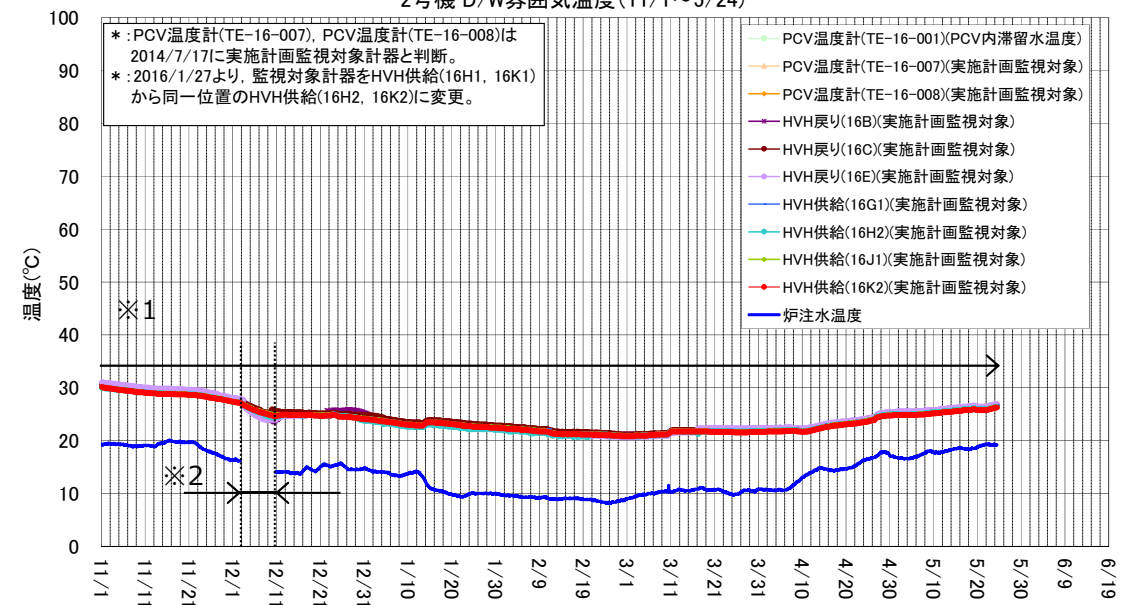
2号機 D/W雰囲気温度(11/1~5/24)
