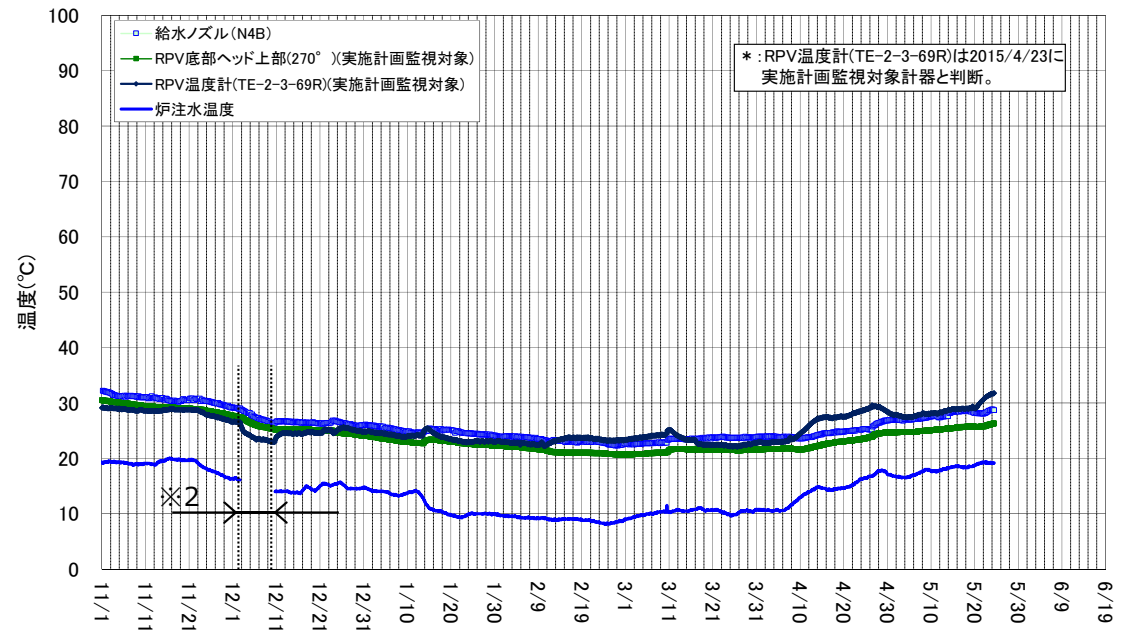
2号機 原子炉圧力容器まわり温度(11/1~5/24)
