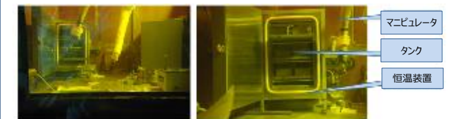
ホットセル内の準備されたサーモスタット装置ユニットの設置
