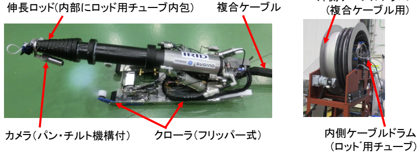
図1 アクセス・調査装置とケーブルドラム
