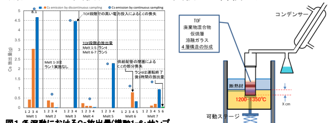
図1 各溶融におけるCs放出量(横軸1-6: サンプル番号、Melt: 溶融試験) 図2 溶融終盤の加熱試験の温度勾配炉とCs捕集装置
