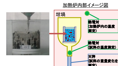
図4 中性子吸収材の乾燥試験
