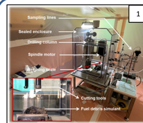
気密室(写真①)における、コアボーリング前の模擬燃料デブリへの飛散抑制材塗布(写真②)。塗布材の飛散抑制効果評価のための気中飛散粒子生成物の監視(写真③)。
