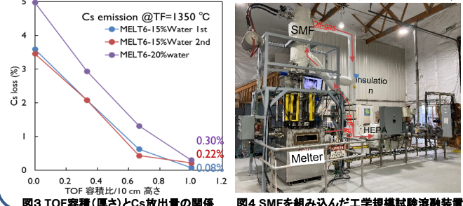
図3 TOF容積(厚さ)とCs放出量の関係 図4 SMFを組み込んだ工学規模試験溶融装置
