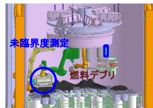
図3 燃料デブリ取り出し時の臨界近接監視
