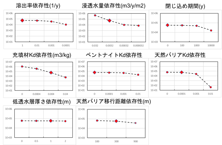
図6 感度構造評価の例（対象処分概念：中深度処分、対象核種：C-14）
