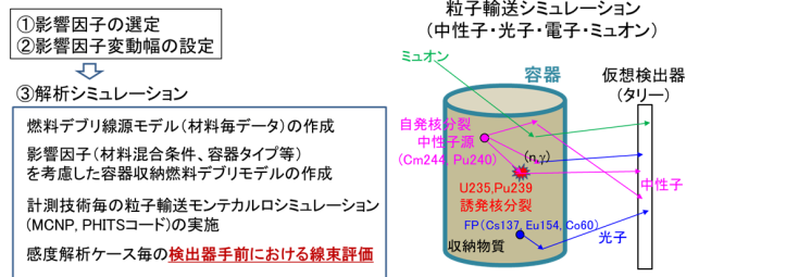
図1 解析シミュレーション（全体の流れ）
