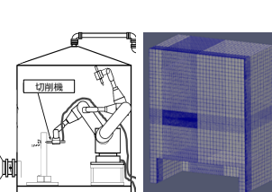
図4 廃炉ハンドブック飛散率測定試験の数値解析
