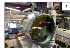
専用施設での空力及び水圧による応力、機械的切削によるダスト再浮遊試験実施(写真④)。
