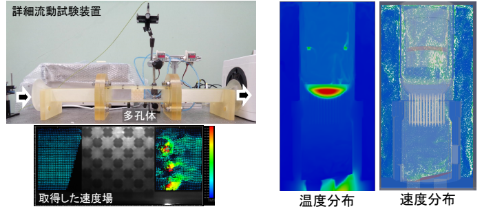
図2 詳細流動試験装置により取得したデータ
