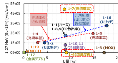
図2 パッシブガンマ線の解析例（Eu-154（1.27MeV）の線束）
