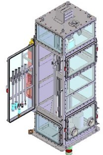
図9 セシウム吸着塔からの試料採取装置
