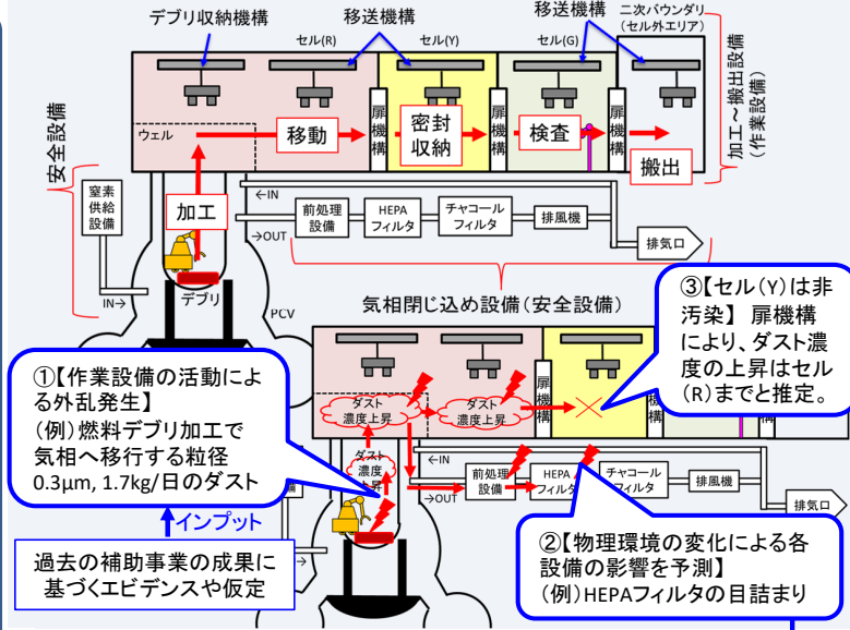
図1 気相閉じ込め設備を再現した場合のデブリ取り出しモデル（※3）
