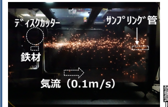
図3 パラメータ試験装置試作機での予備試験(光点は鉄の切削ダスト)
