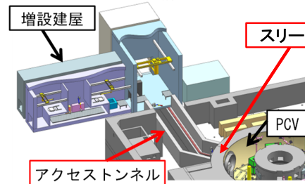
図3 アクセストンネルイメージ
