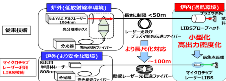
図5 光ファイバーLIBSの基本型と長尺化技術
