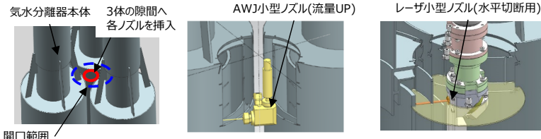
図1 気水分離器本体部の切断イメージ(AWJ切断、レーザ切断)
