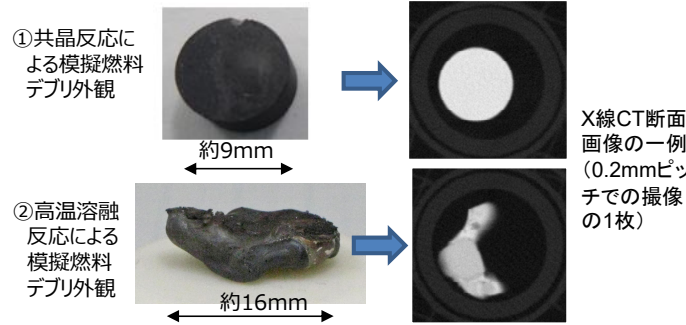
図1 調製した模擬燃料デブリとX線CT撮像の例
