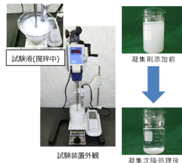
図2 RO濃縮水処理試験
