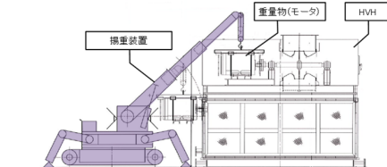
図5 HVH解体用揚重装置イメージ
