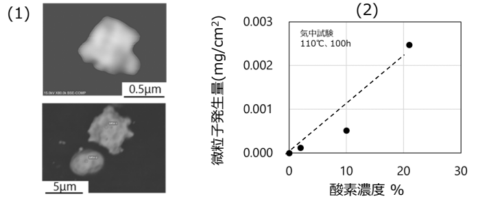
図1 Zr(O)+ (U,Zr)O_2 の気中試験で発生した微粒子の(1)電子顕微鏡写真、(2)微粒子発生量の酸素濃度依存性
