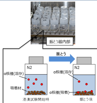
図1 \alpha 核種吸着試験
