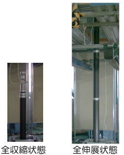
図3 3段テレスコピックによる簡易試験
