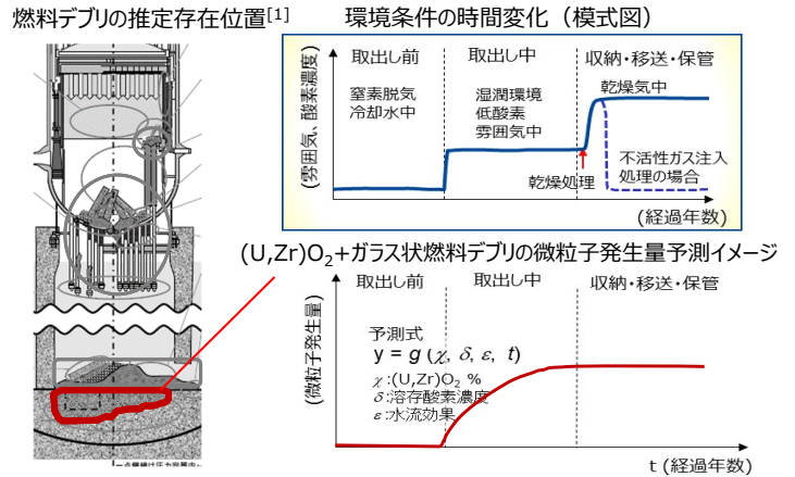
図2 燃料デブリの廃炉工程における微粒子発生量の推定方針案を示す模式図
