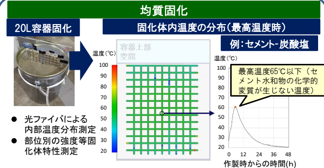
図1 ALPSスラリー(模擬物)のセメント均質固化試験における固化体内温度
