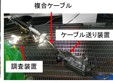
図3 ケーブル送り装置での送り状況
