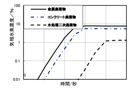
図1 水素発生速度の評価モデル（ラジオリシスモデル）イメージ図
