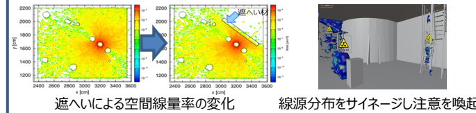
図2 線源・線量率推定結果の可視化例
