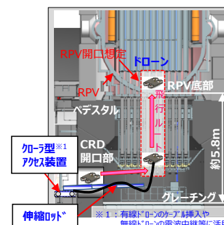
図2 ドローンによるアクセスイメージ
