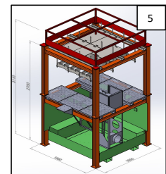
飛散抑制材適用性確認試験のためのモックアップ設備(図⑤)。
