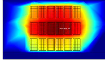
図4 200ℓドラム缶の集積配置による温度分布解析結果（セメント固化体、放射能濃度 1 \times 10^9 Bq）
