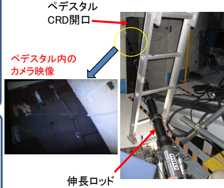
図2 ペDESTル内の調査状況
