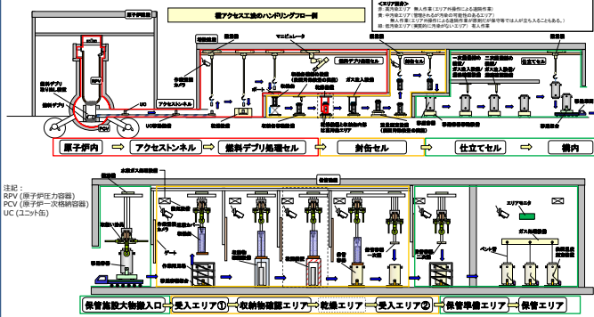
図1 粒状・塊状の燃料デブリの一連の取り扱いプロセス例
