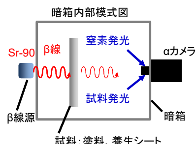
図2 アルファカメラのβ線源による発光試験
