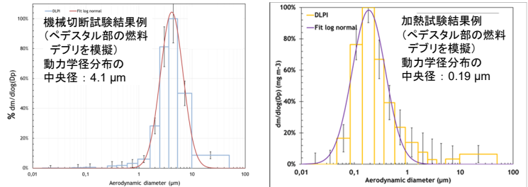
図1 生成した微粒子の動力学径分布の測定例
