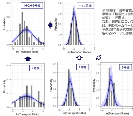
図8 汚染濃度分布の号機による違いに関する解析例
