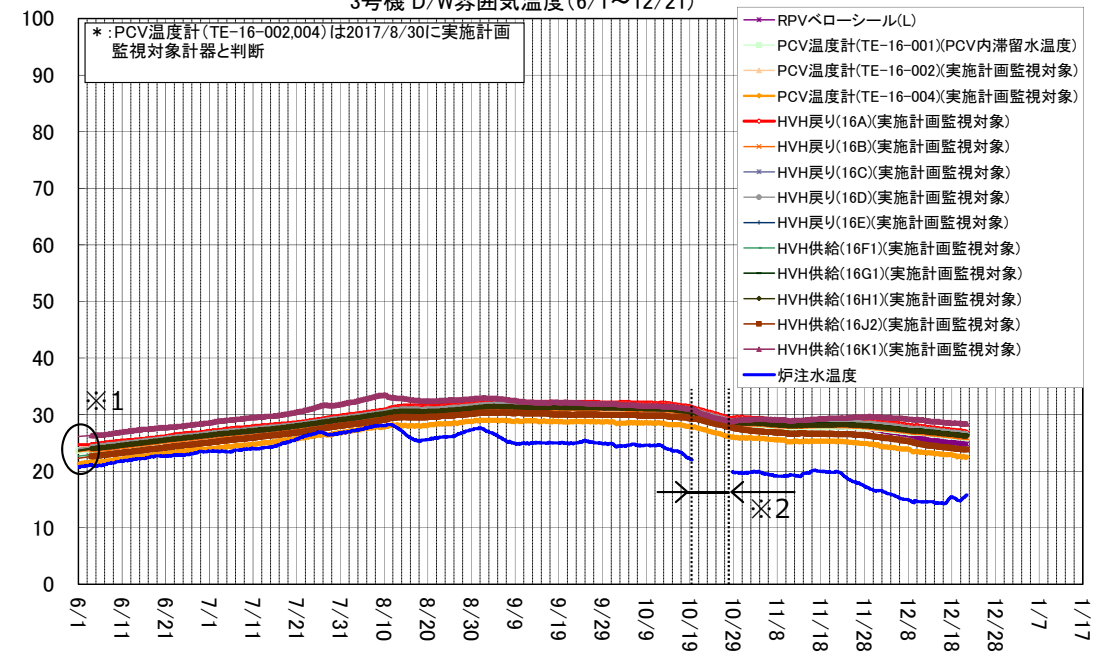
3号機 D/W雰囲気温度 (6/1~12/21)
