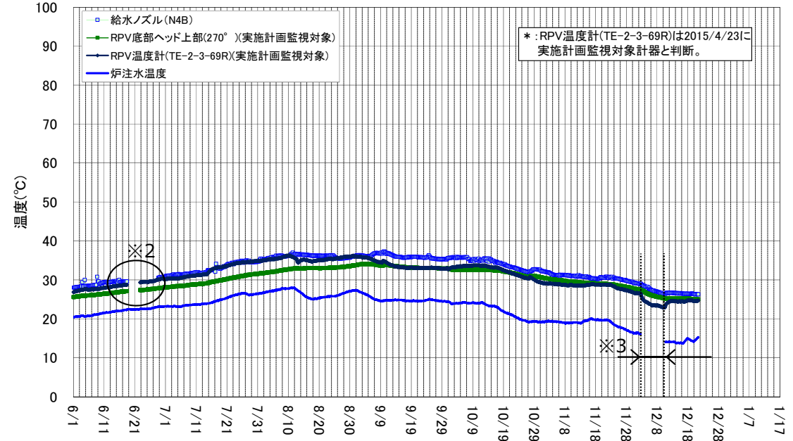
2号機 原子炉压力容器まわり温度(6/1~12/21)
