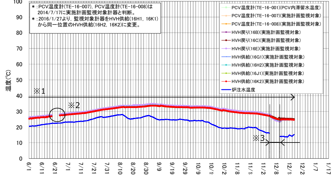
2号機 D/W雰囲気温度(6/1~12/21)
