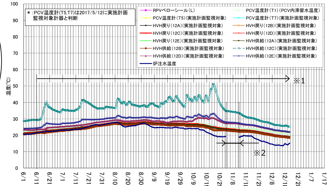
1号機 D/W雰囲気温度(6/1~12/21)
