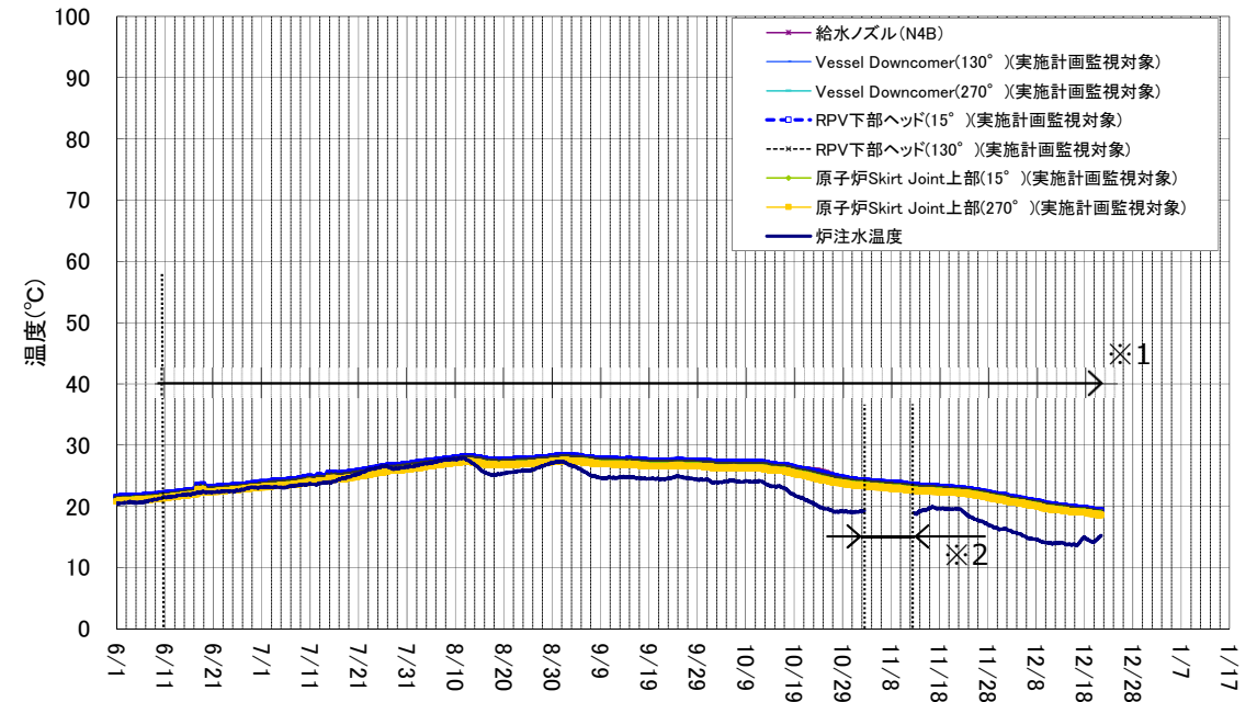
1号機 原子炉压力容器まわり温度(6/1~12/21)
