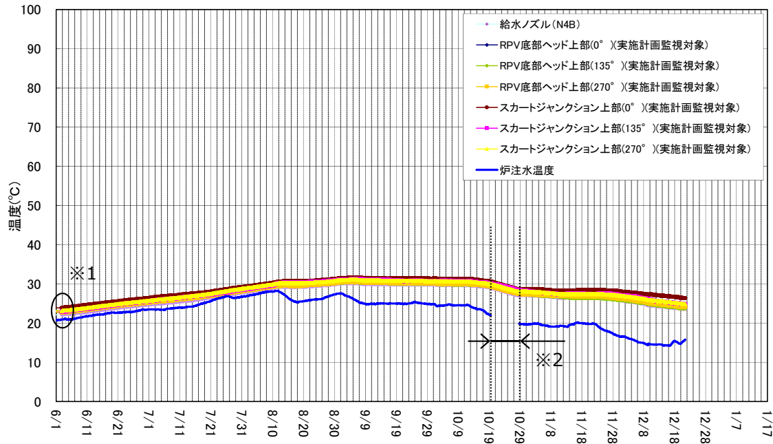
3号機 原子炉压力容器まわり温度 (6/1~12/21)
