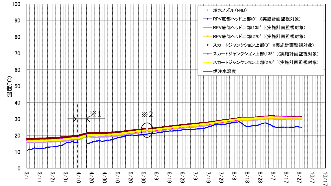
3号機 原子炉圧力容器まわり温度 (3/1～9/28)
