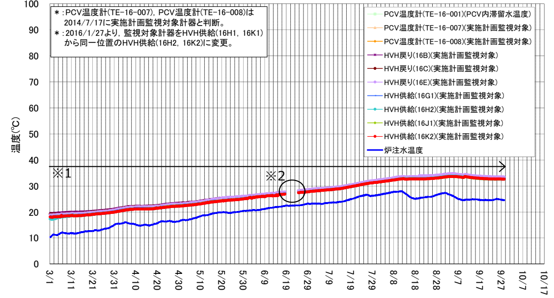
2号機 D/W雰囲気温度 (3/1～9/28)
