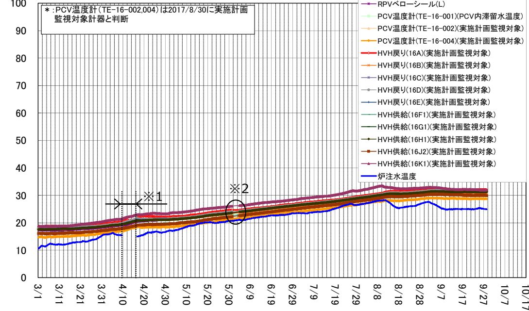
3号機 D/W雰囲気温度 (3/1～9/28)
