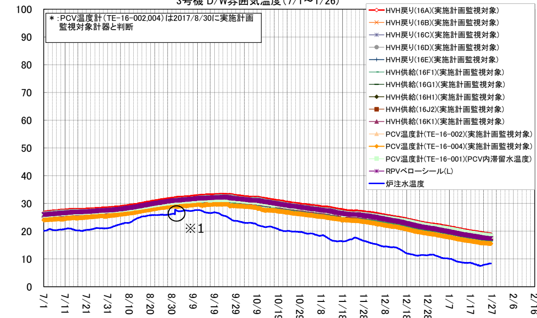
3号機 D/W雰囲気温度(7/1~1/26)
