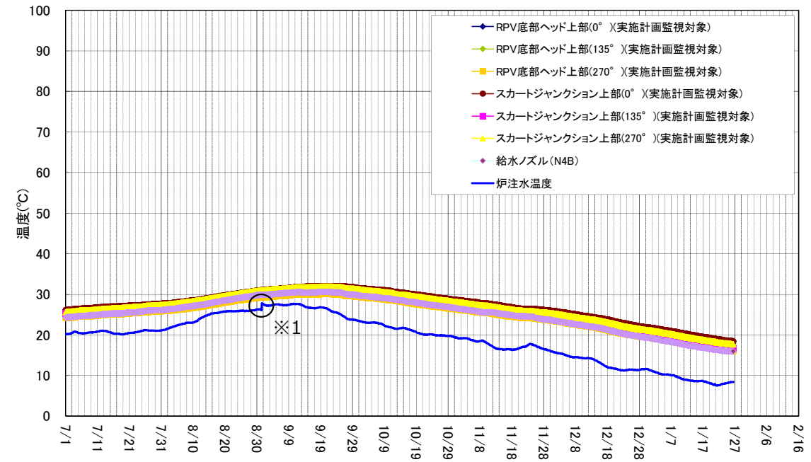
3号機 原子炉压力容器まわり温度(7/1~1/26)
