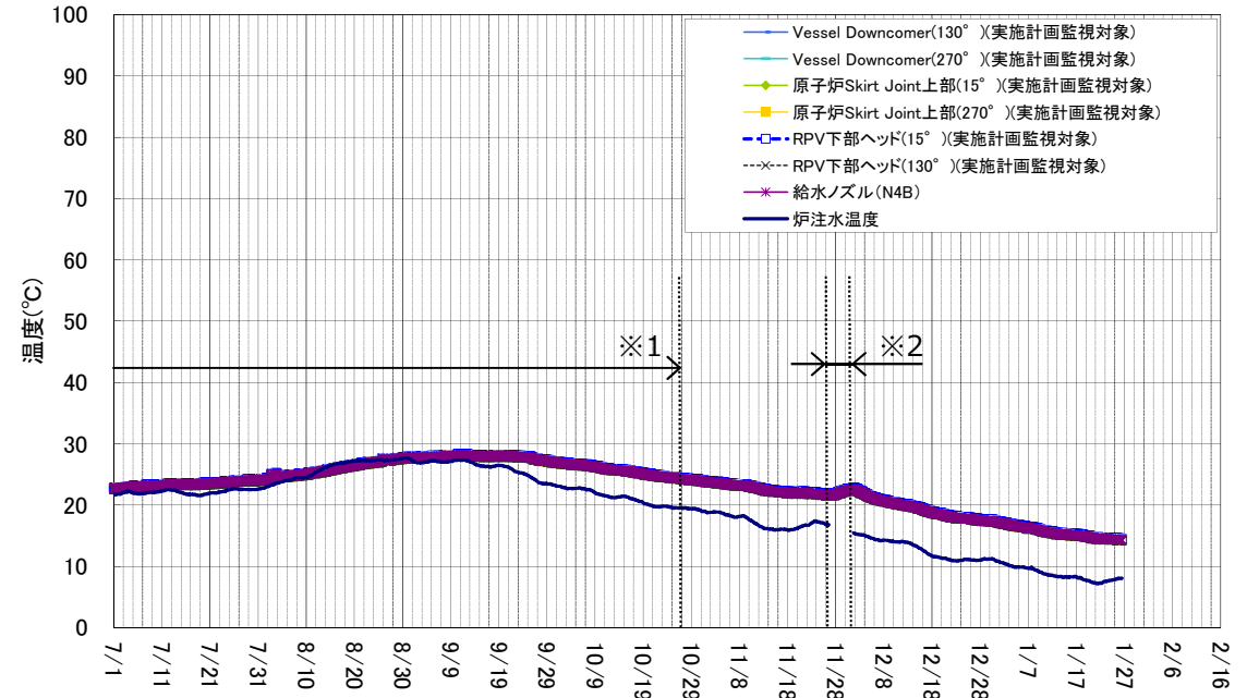
1号機 原子炉圧力容器まわり温度(7/1~1/26)
