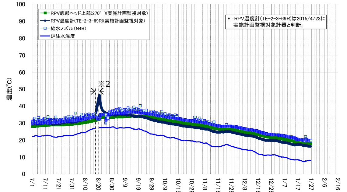
2号機 原子炉圧力容器まわり温度 (7/1~1/26)
