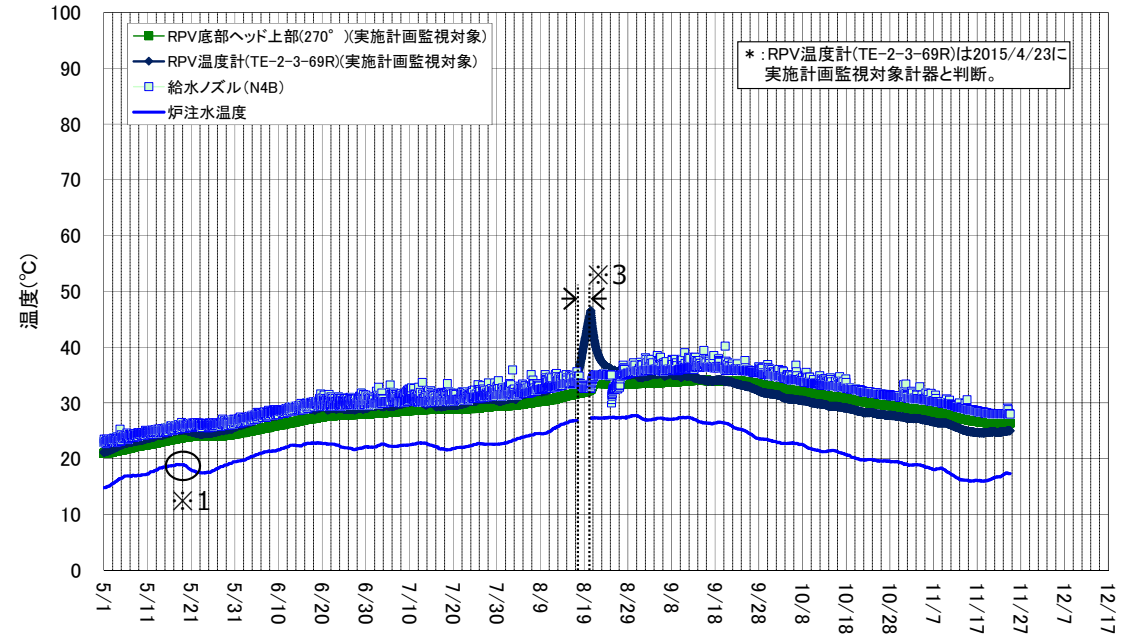
2号機 原子炉圧力容器まわり温度(5/1~11/24)
