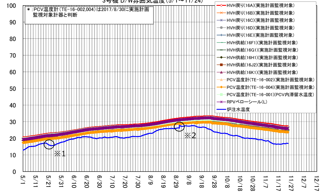
3号機 D/W雰囲気温度(5/1~11/24)
