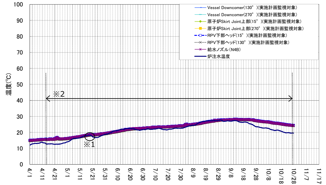
1号機 原子炉压力容器まわり温度(4/1~10/27)
