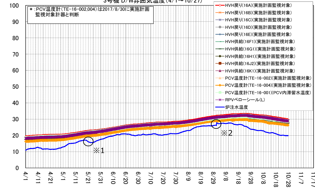
3号機 D/W雰囲気温度(4/1~10/27)
