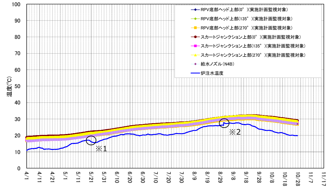
3号機 原子炉压力容器まわり温度(4/1~10/27)
