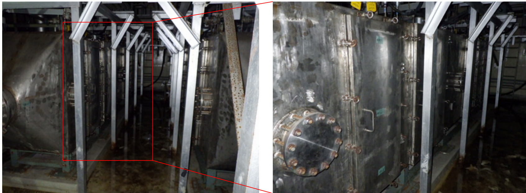
4号機SGTSフィルタトレインの様子
