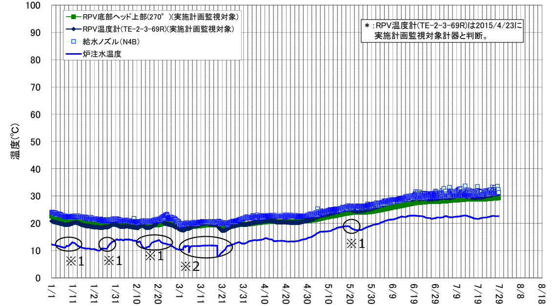
2号機 原子炉圧力容器まわり温度(1/1~7/28)
