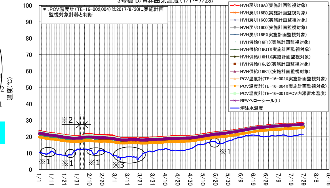
3号機 D/W雰囲気温度(1/1~7/28)
