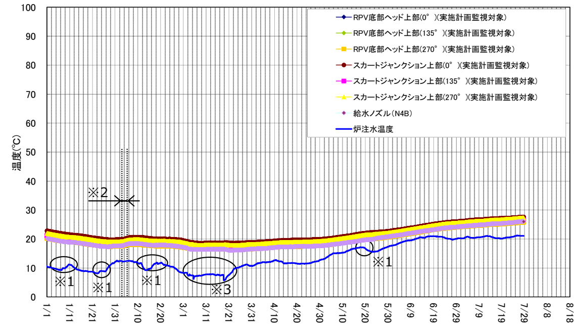
3号機 原子炉压力容器まわり温度(1/1~7/28)
