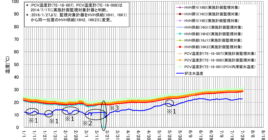
2号機 D/W雰囲気温度(1/1~7/28)
