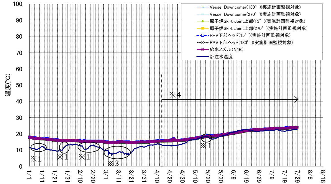
1号機 原子炉圧力容器まわり温度(1/1~7/28)
