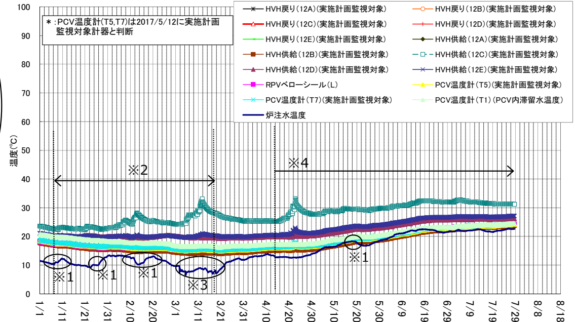
1号機 D/W雰囲気温度(1/1~7/28)
