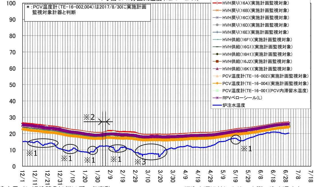
3号機 D/W雰囲気温度(12/1~6/30)
