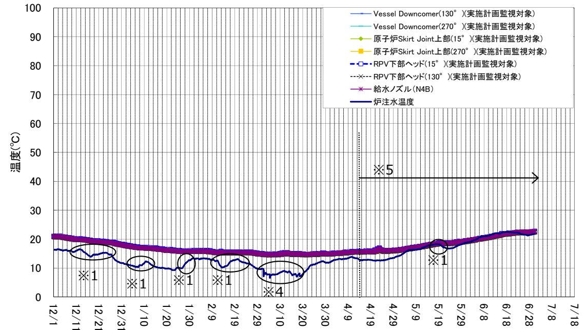
1号機 原子炉圧力容器まわり温度(12/1~6/30)
