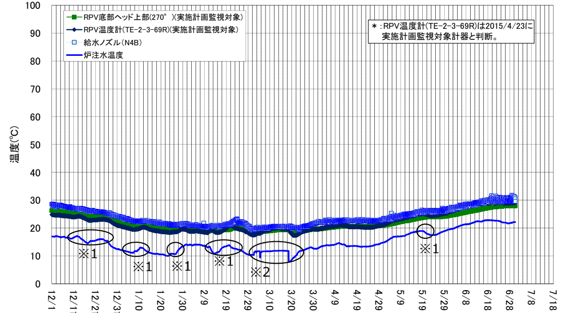
2号機 原子炉圧力容器まわり温度 (12/1~6/30)
