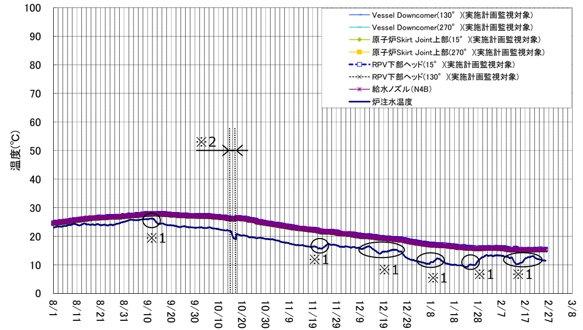
1号機 原子炉圧力容器まわり温度(8/1~2/25)
