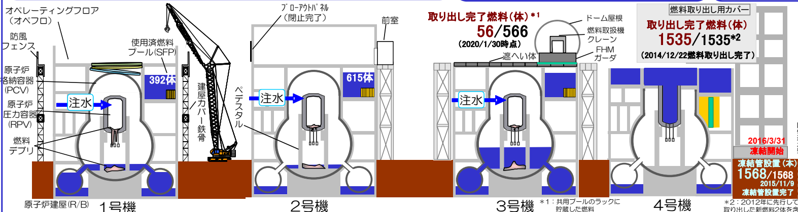
<ガレキ落下防止・緩和対策の全体概要> ● Xプレス撤去箇所
