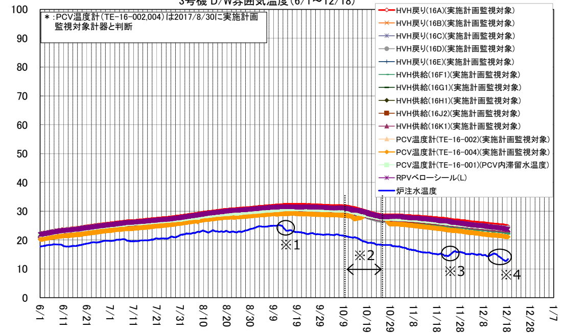
3号機 D/W雰囲気温度(6/1~12/18)
