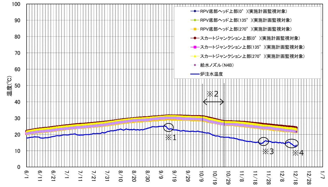
3号機 原子炉压力容器まわり温度(6/1~12/18)
