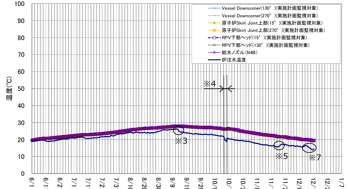
1号機 原子炉压力容器まわり温度(6/1~12/18)
