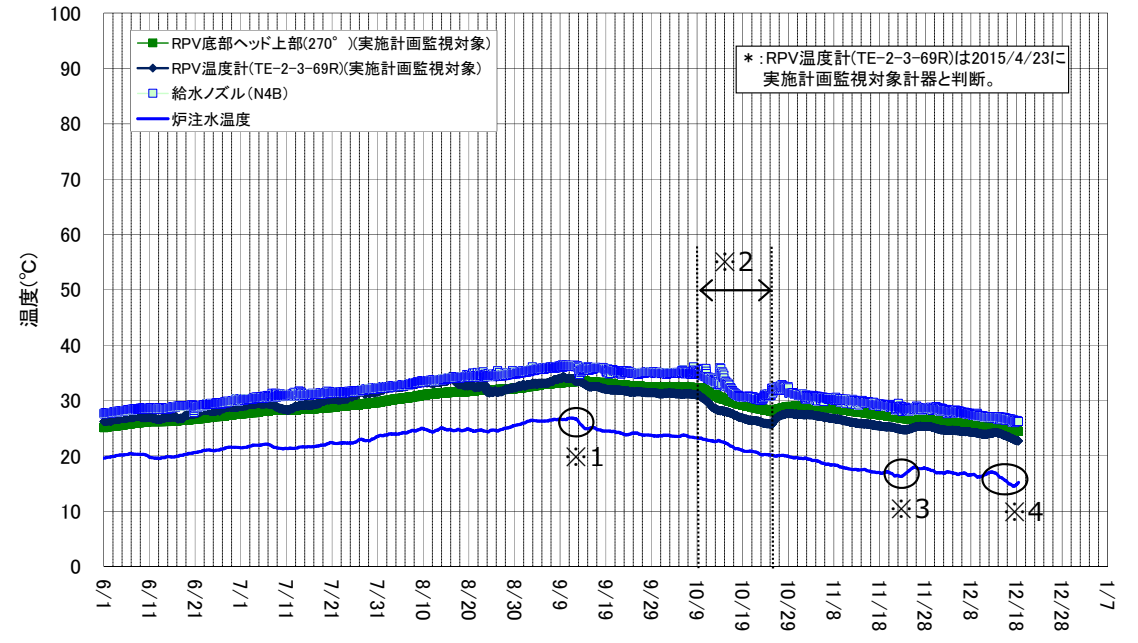
2号機 原子炉压力容器まわり温度(6/1~12/18)
