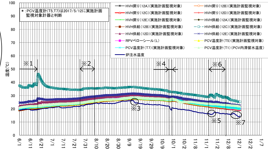
1号機 D/W雰囲気温度(6/1~12/18)
