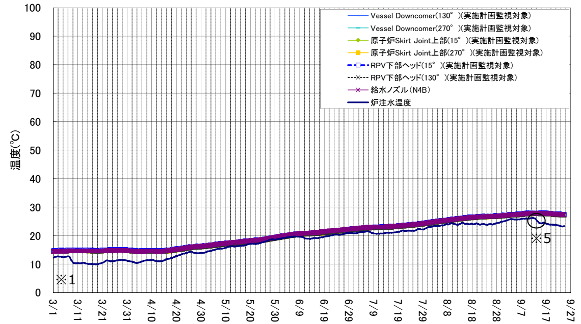
1号機 原子炉圧力容器まわり温度(3/1~9/24)
