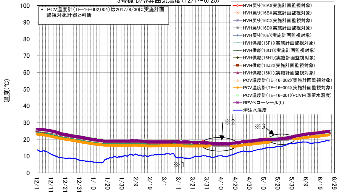
3号機 D/W雰囲気温度(12/1~6/25)
