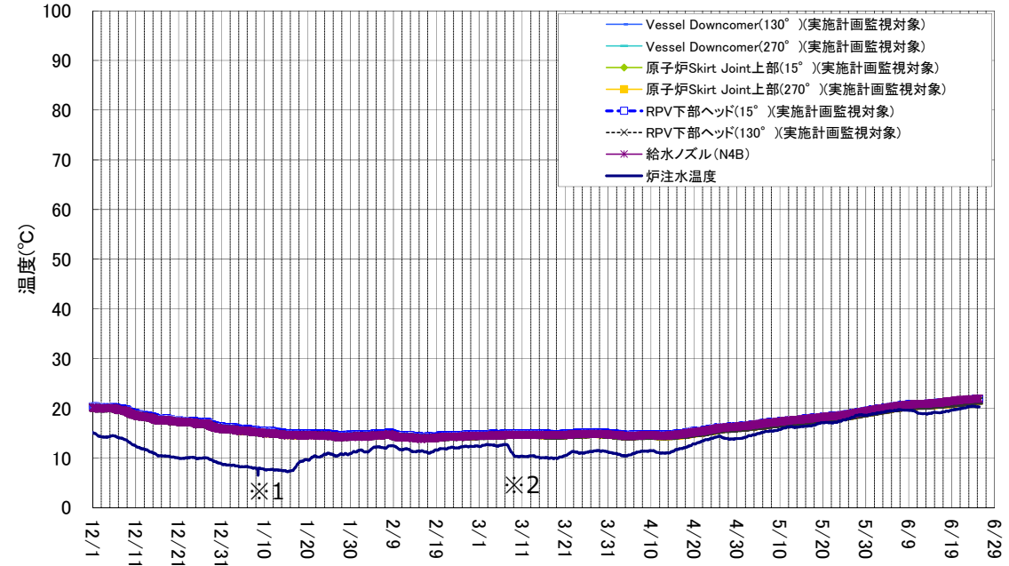
1号機 原子炉压力容器まわり温度 (12/1~6/25)
