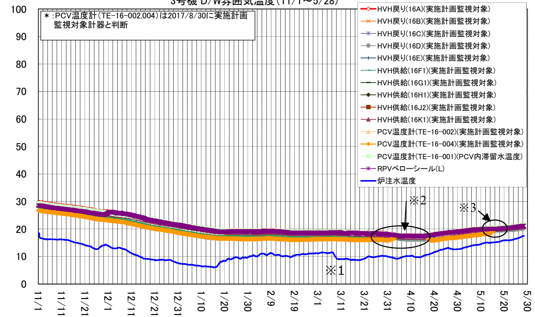
3号機 D/W雰囲気温度(11/1~5/28)
