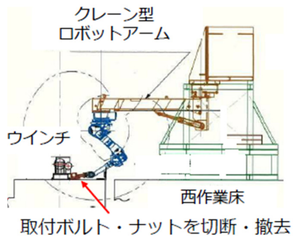
ウインチ撤去
