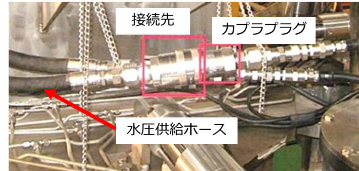
図1 水圧供給用ホース接続イメージ
