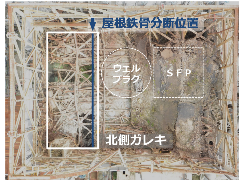
屋根鉄骨分断位置（予定）
