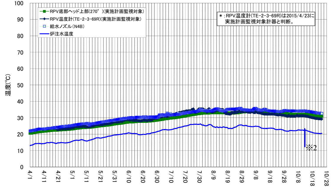
2号機 原子炉压力容器まわり温度 (4/1~10/24)
