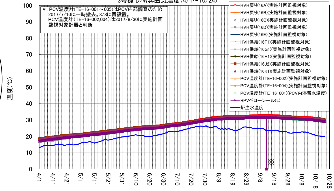
3号機 D/W雰囲気温度(4/1~10/24)
