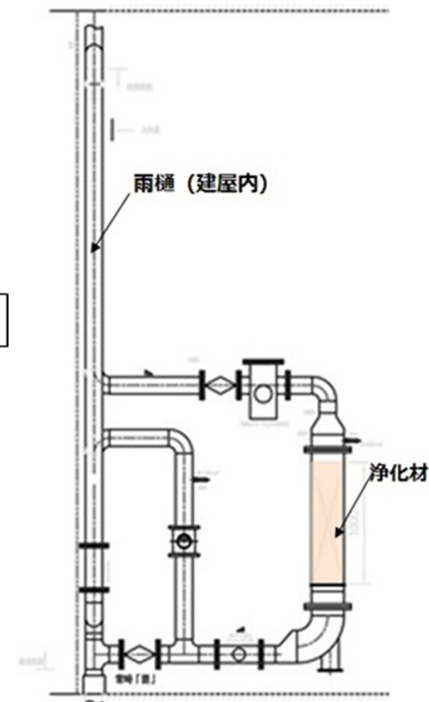
図2 雨水浄化装置 (イメージ図)
