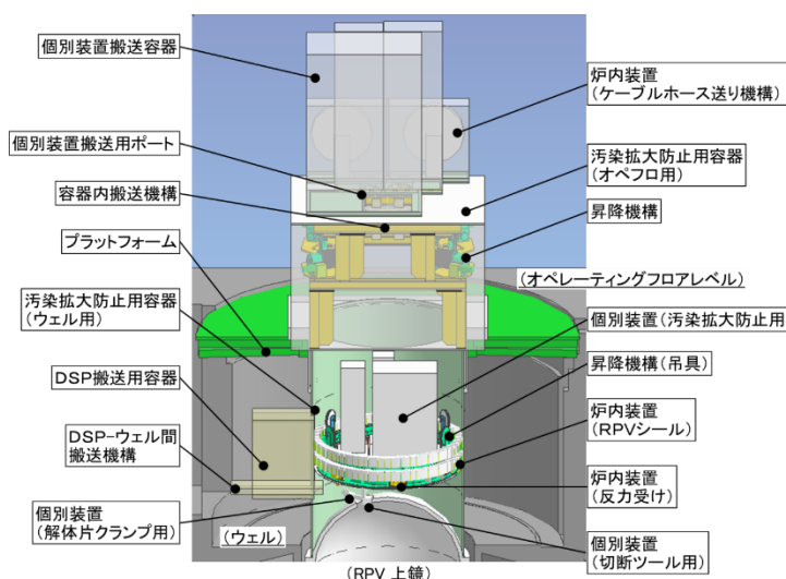
炉内装置全体構成図 (案)
