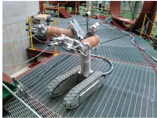
試作機タイプ II (双腕型)
