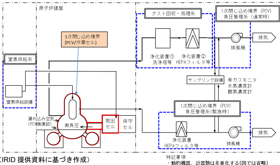
図 4.5-23 1 次閉じ込め境界 (PCV) 用負圧管理システム検討例 (気中一横アクセス工法)
