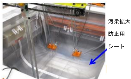
汚染拡大防止用シートの適用性確認試験 (DSP 内)
