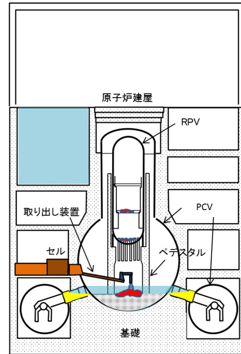
c. 気中-横アクセス工法
