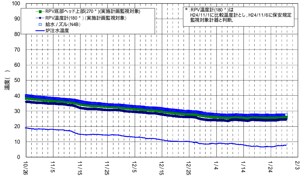
2号機 原子炉压力容器まわり温度 (10/26 ~ 1/29)
