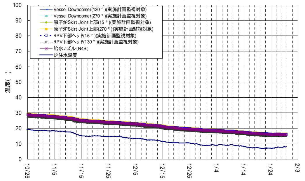
1号機 原子炉压力容器まわり温度 (10/26 ~ 1/29)
